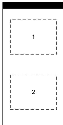
図 4-1. DPY パッケージ、2 ピン DFN1006 (上面図)
