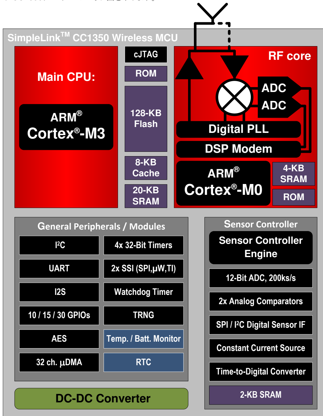
図 1-1. CC1350ブロック図
