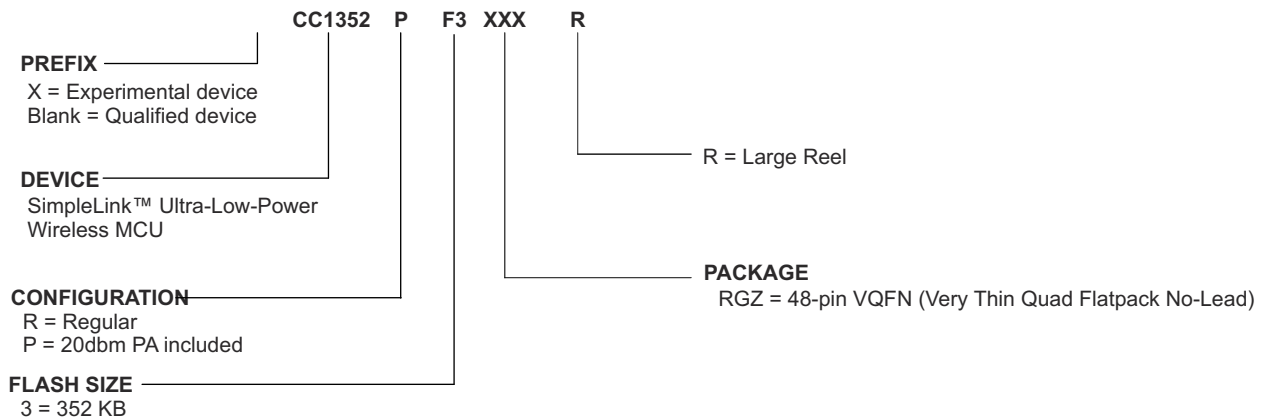
✎ 11-1. Device Nomenclature
