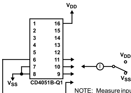
図 6-10. デバイスの静止電流
