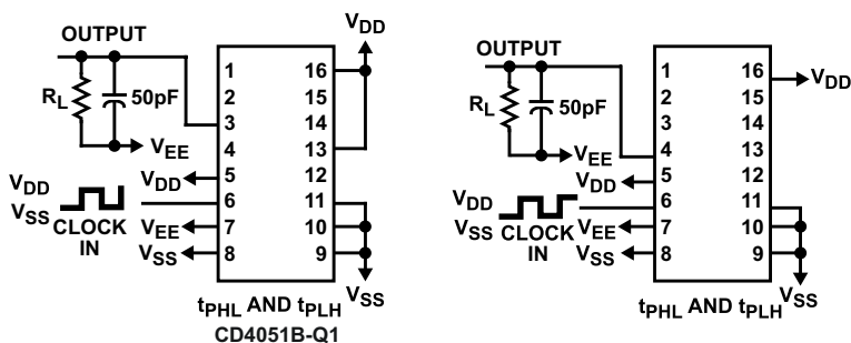
図 6-8. 伝搬遅延 - インビット入力から信号出力
