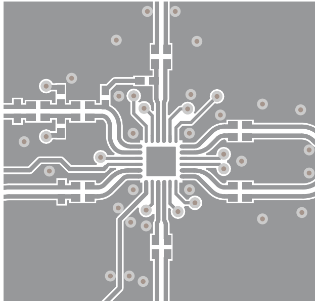
☒ 12-1. Layout Example, Top Layer
