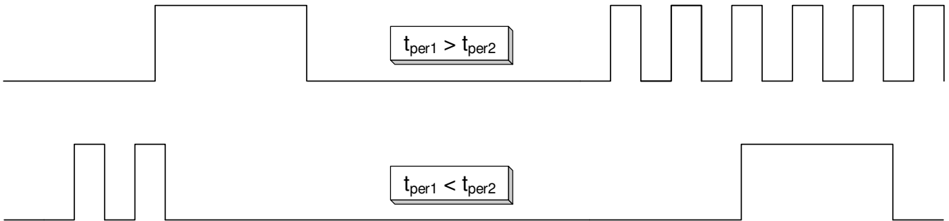
9-8. Glitchless Divider Update
