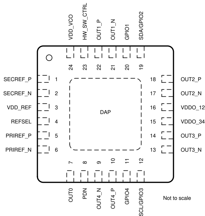
図 6-1. CDCE6214-Q1 RGE Package 24-Pin VQFN Top View
