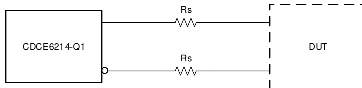
8-14. LP-HCSL Output
