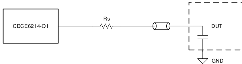
8-11. LVCMOS Output
