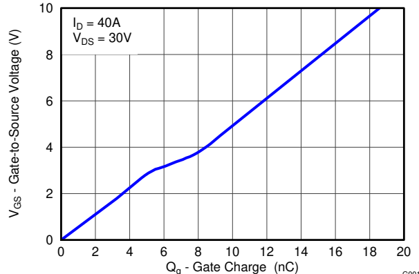
ゲート電荷
