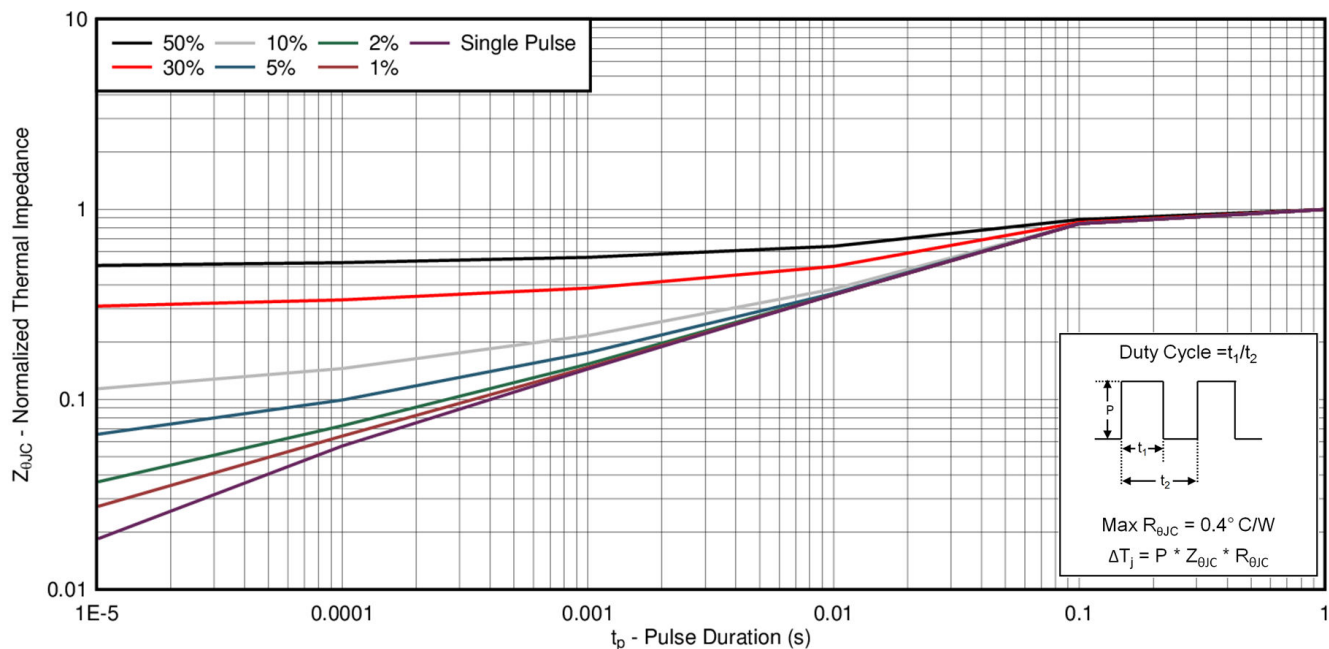
図 3-1. 過渡熱抵抗
