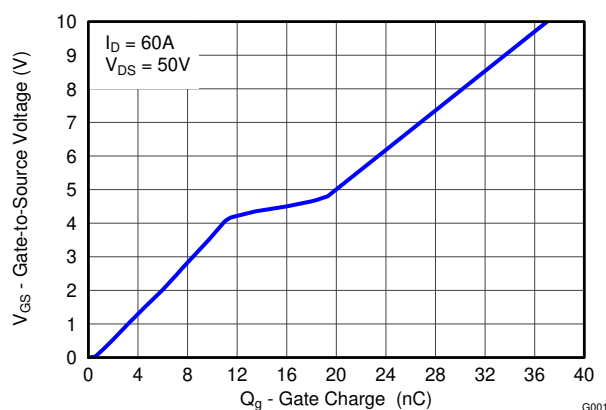
ゲート電荷
