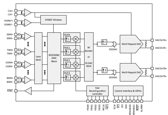
ブロック図
