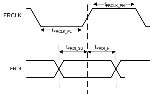
図 6-6. FRDI Timing Diagram
