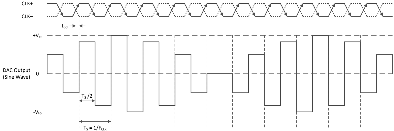
图 7-7. RF Mode Timing Diagram
