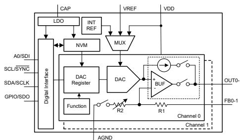
概略ブロック図
