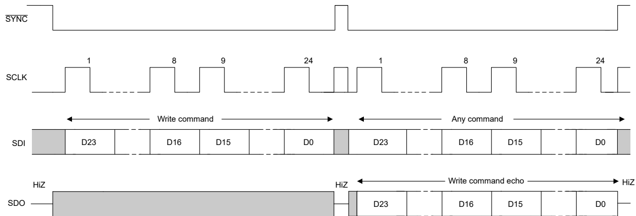
図 7-16. SPI Write Cycle
