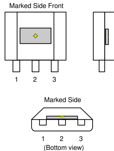
図 9-3. TO-92 (LPG) パッケージ
