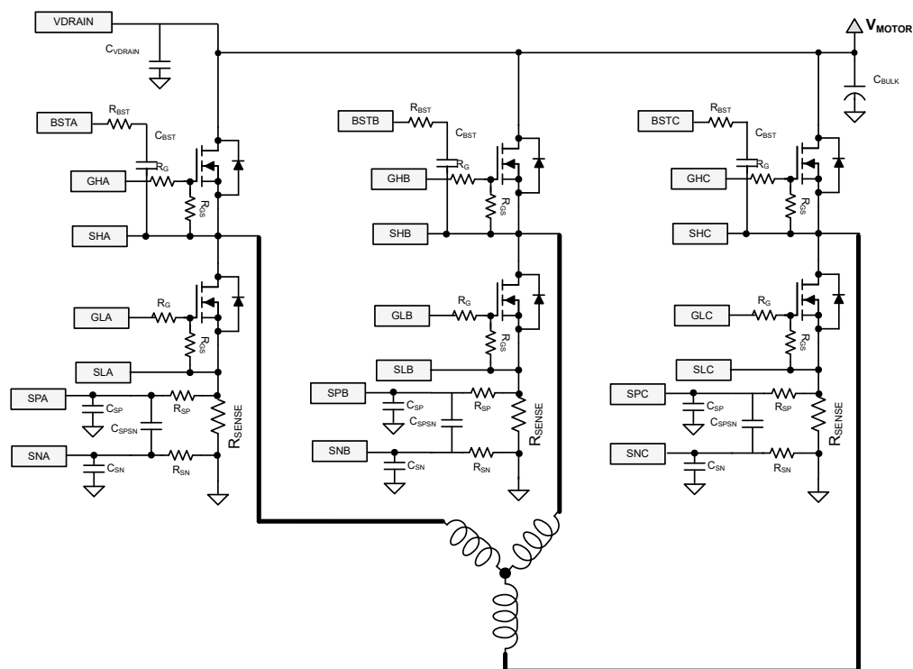
図 7-1. DRV8363 の代表的なアプリケーション回路
