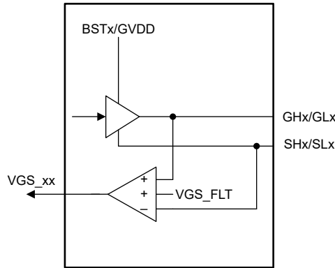
図 6-19. DRV8363 V GS モニタ
