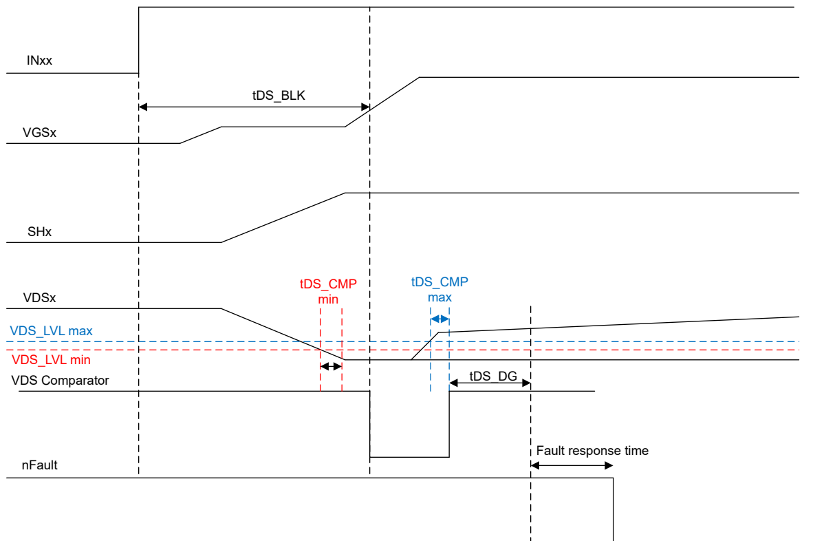
図 6-18. DRV8363 V_{DS} モニタのタイミング
