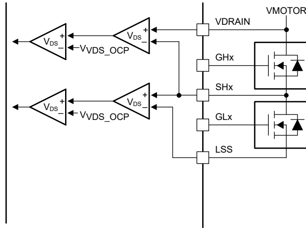
図 6-17. DRV8363 V_{DS} モニタ
