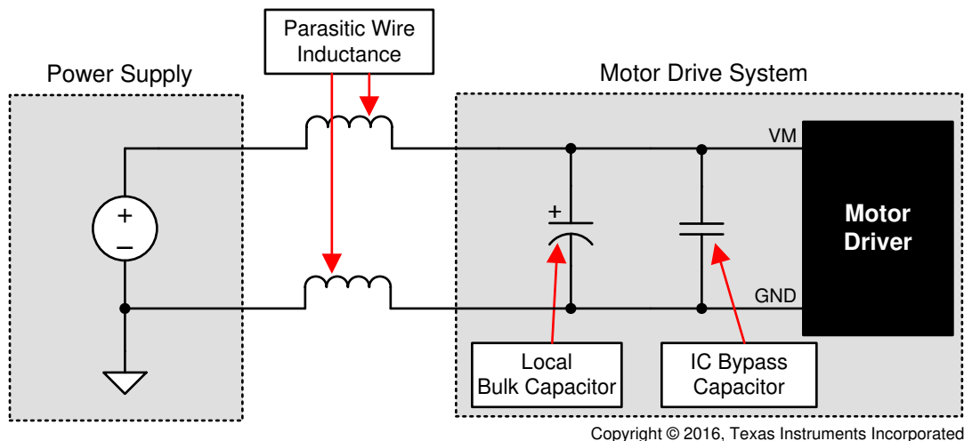
図 7-16. 外部電源を持つシステムの構成例
