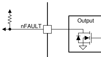
図 6-12. nFAULT ピン
