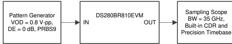
图 11. Minimal Rx/Tx Channel Test Setup
