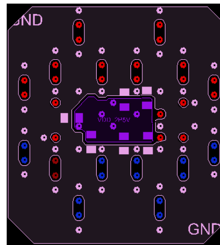
☒ 32. Bottom Layer
