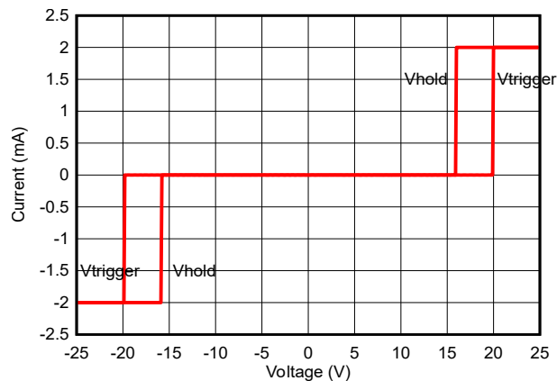
図 5-2. DC I-V Curve
