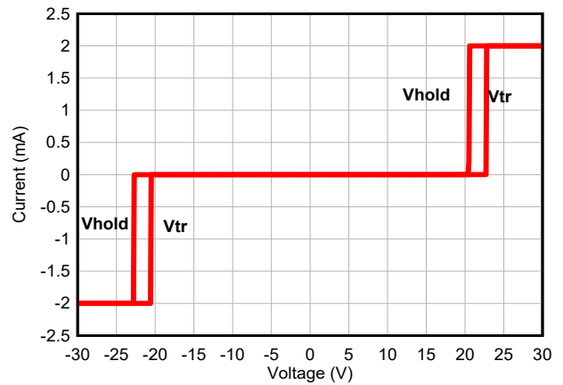
図 5-4. DC Voltage Sweep I-V Curve
