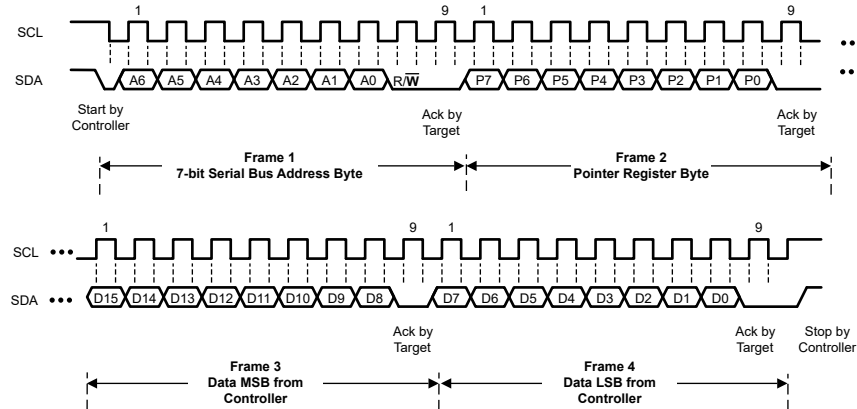
6-4. Write Frame
