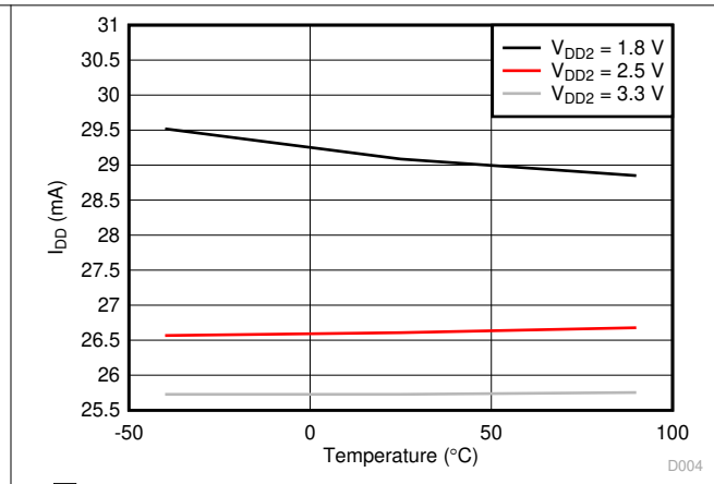
7-2. Dynamic IDD1 vs. Ambient Temperature
