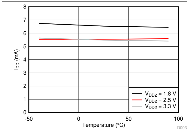
7-1. Static IDD1 vs. Ambient Temperature
