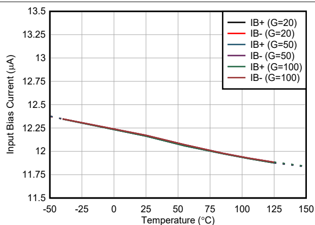
図 5-12. 入力バイアス電流と温度との関係
