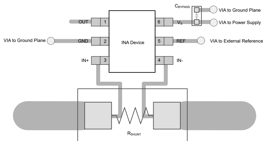
図 7-3. INA187-Q1 SOT-23 6 ピン (DBV) パッケージの推奨レイアウト
