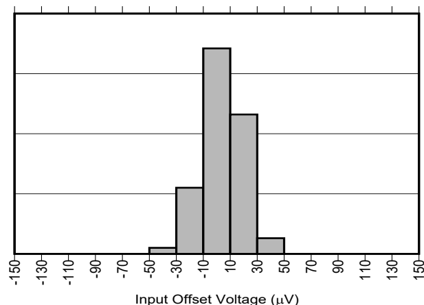
図 5-1. INA299 入力オフセット電圧の製品分布
