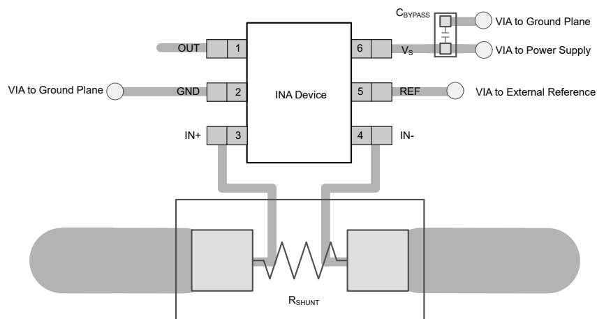
図 7-3. INA299 SOT-23 6 ピン (DBV) パッケージの推奨レイアウト
