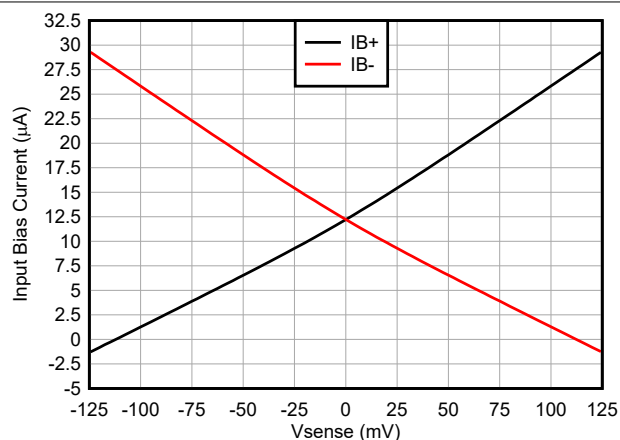
図 5-13. INA299 ゲイン = 20V/V、入力バイアス電流と V_{\text{SENSE}} との関係
