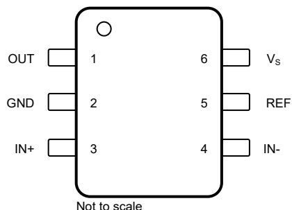
図 4-1. INA299 : DBV パッケージ 6 ピン SOT-23 上面図
