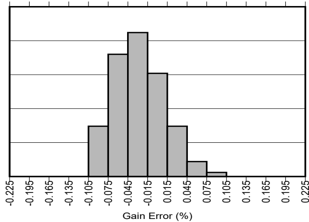
図 5-7. INA299 ゲイン誤差の製品分布
