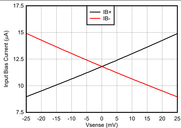
図 5-15. INA299 ゲイン = 100V/V 入力バイアス電流と V_{\text{SENSE}} との関係
