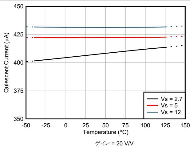
図 5-25. 静止電流と温度との関係
