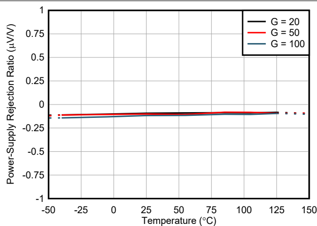
図 5-9. 電源除去比と温度との関係
