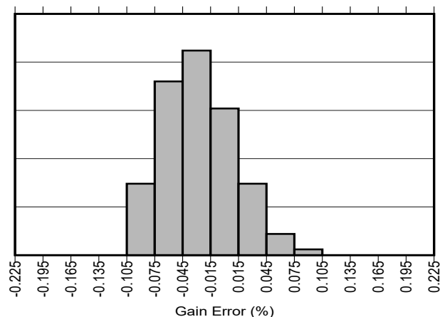
図 5-7. INA299-Q1 ゲイン誤差の製品分布
