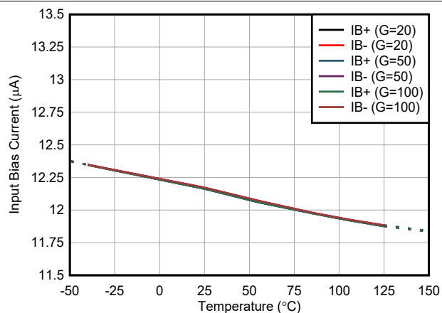
図 5-12. 入力バイアス電流と温度との関係
