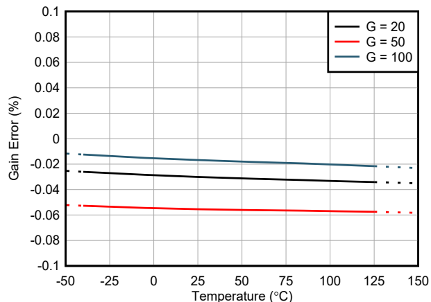
図 5-8. ゲイン誤差と温度との関係
