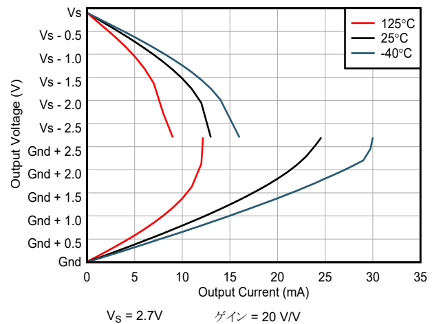
図 5-16. 出力電圧と出力電流との関係
