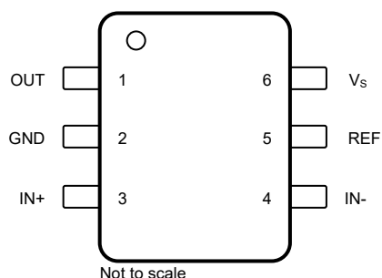
図 4-1. INA299-Q1 : DBV パッケージ 6 ピン SOT-23 上面図
