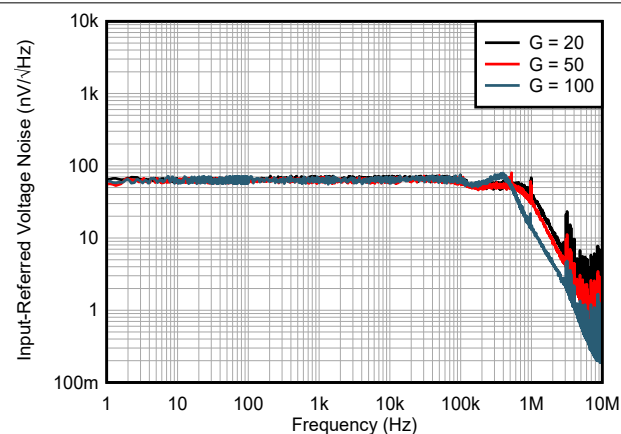
図 5-22. 入力換算ノイズと周波数との関係
