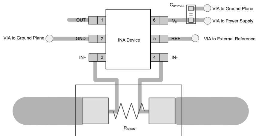
図 7-3. INA299-Q1 SOT-23 6 ピン (DBV) パッケージの推奨レイアウト
