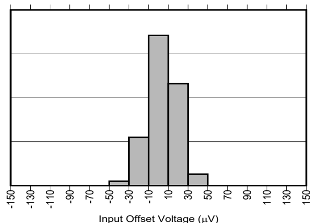
図 5-1. INA299-Q1 入力オフセット電圧の製品分布
