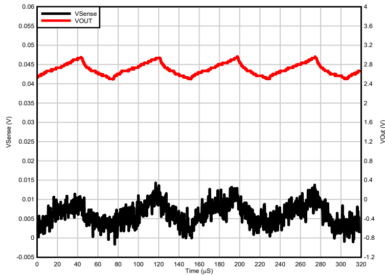
図 7-2. ハイサイド モーター電流測定
