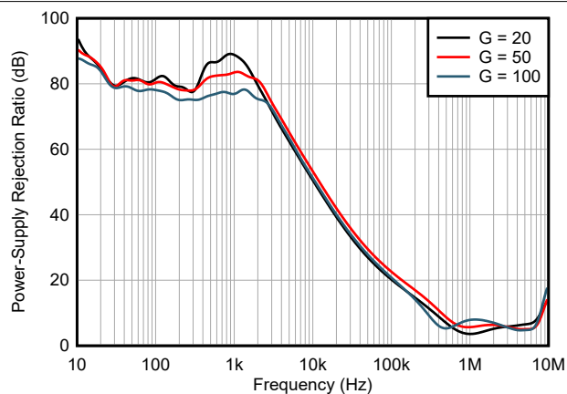
図 5-10. 電源除去比と周波数との関係
