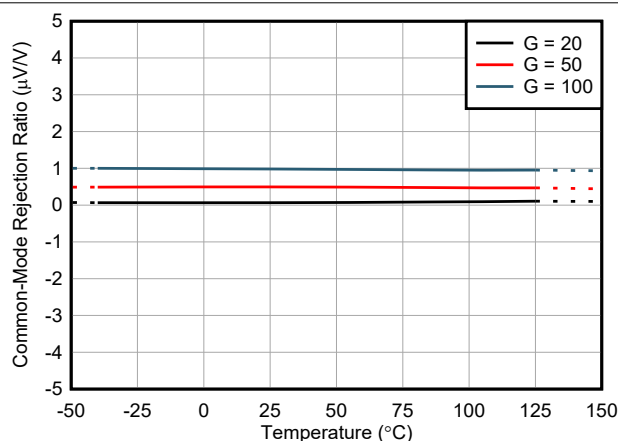
図 5-4. 同相除去比と温度との関係
