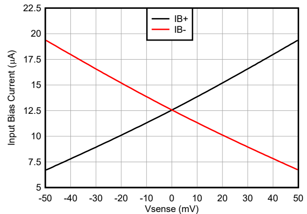
図 5-14. INA299-Q1 ゲイン = 50V/V、入力バイアス電流と V_{\text{SENSE}} との関係
