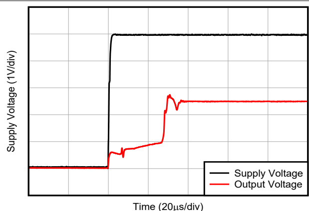
図 5-31. スタートアップ応答
