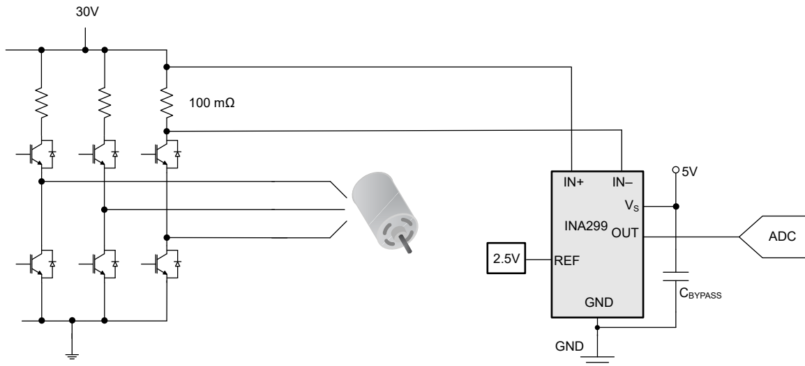
図 7-1. ハイサイド モーター電流センシング アプリケーション回路
