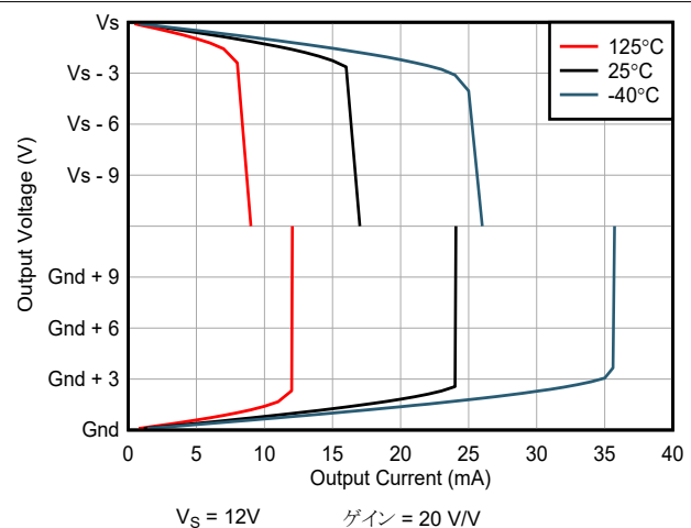
図 5-18. 出力電圧と出力電流との関係
