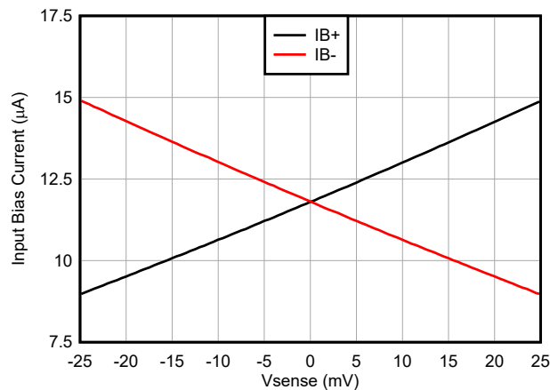
図 5-15. INA299-Q1 ゲイン = 100V/V 入力バイアス電流と V_{\text{SENSE}} との関係
