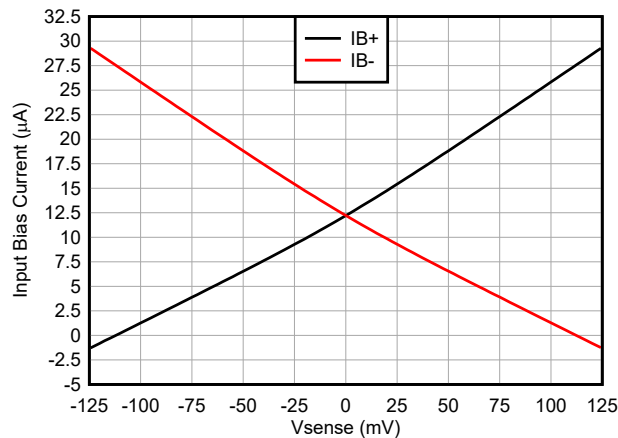
図 5-13. INA299-Q1 ゲイン = 20V/V、入力バイアス電流と V_{\text{SENSE}} との関係
