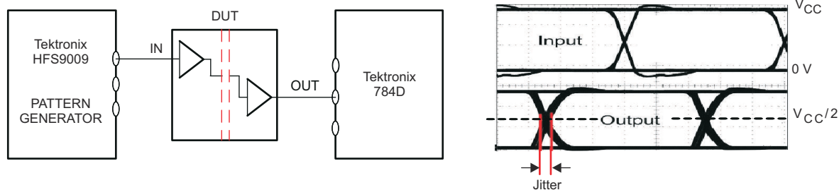
図 6-4. ピーク ツー ピーク アイパターン ジッタ テスト回路と電圧波形
