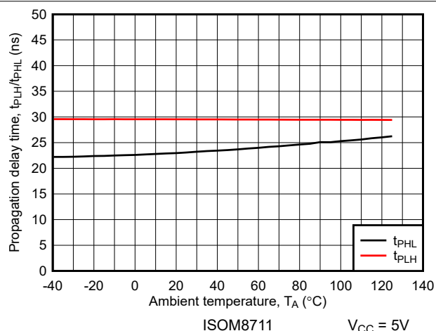
図 6-22. 伝搬遅延時間と周囲温度との関係
