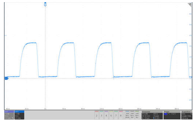
図 9-7. I_F = 6\text{mA} での標準出力波形
