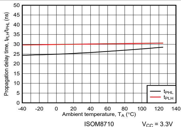
図 6-19. 伝搬遅延時間と周囲温度との関係
