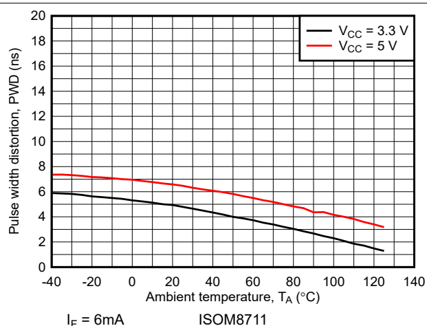
図 6-24. パルス幅歪みと周囲温度との関係
