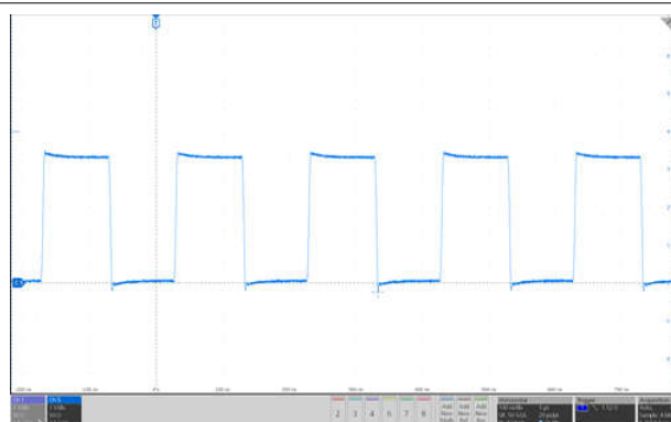
図 9-2. I_F = 2mA での標準出力波形
