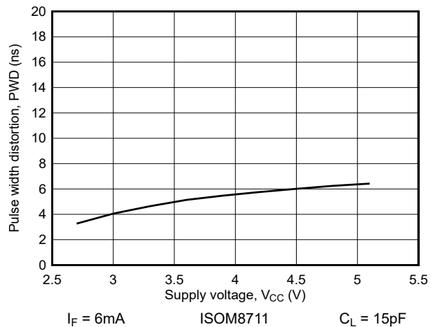
図 6-26. パルス幅歪みと電源電圧との関係
