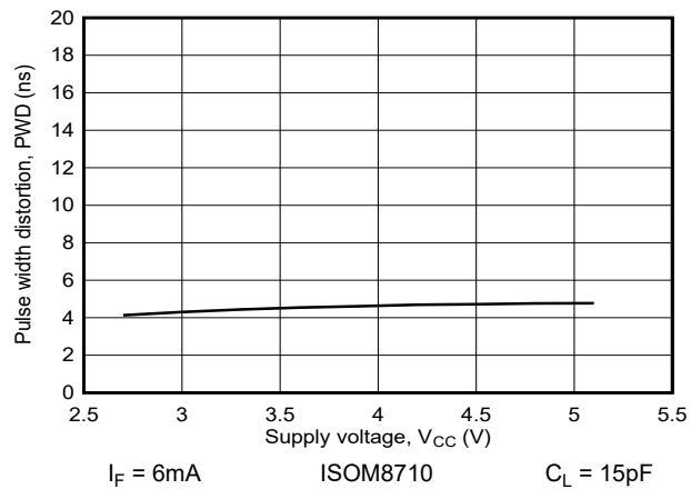
図 6-25. パルス幅歪みと電源電圧との関係
