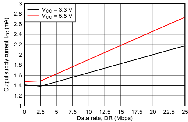
図 6-13. 出力電源電流とデータ レートとの関係
