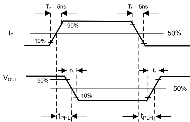
図 7-4. スwitchング タイミング波形
