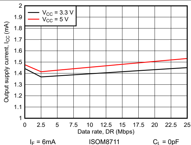
図 6-12. 出力電源電流とデータ レートとの関係
