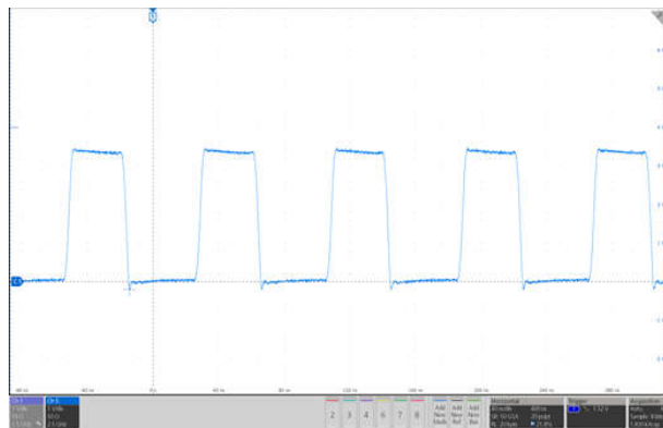
図 9-6. I_F = 6\text{mA} での標準出力波形
