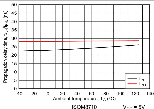
図 6-21. 伝搬遅延時間と周囲温度との関係
