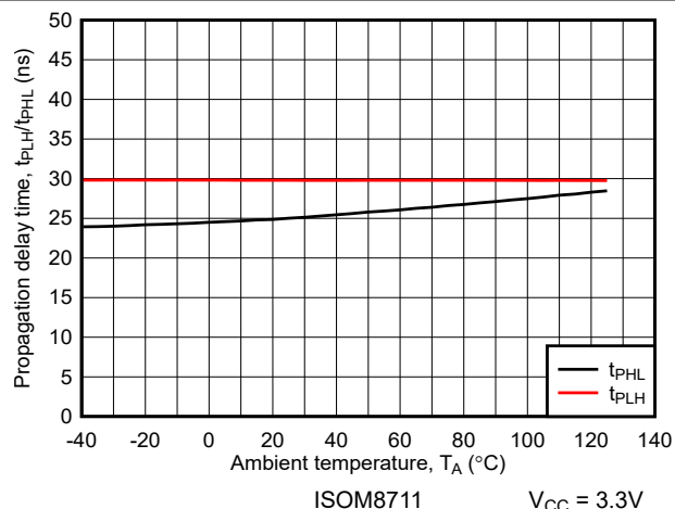
図 6-20. 伝搬遅延時間と周囲温度との関係
