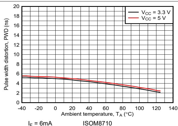
図 6-23. パルス幅歪みと周囲温度との関係
