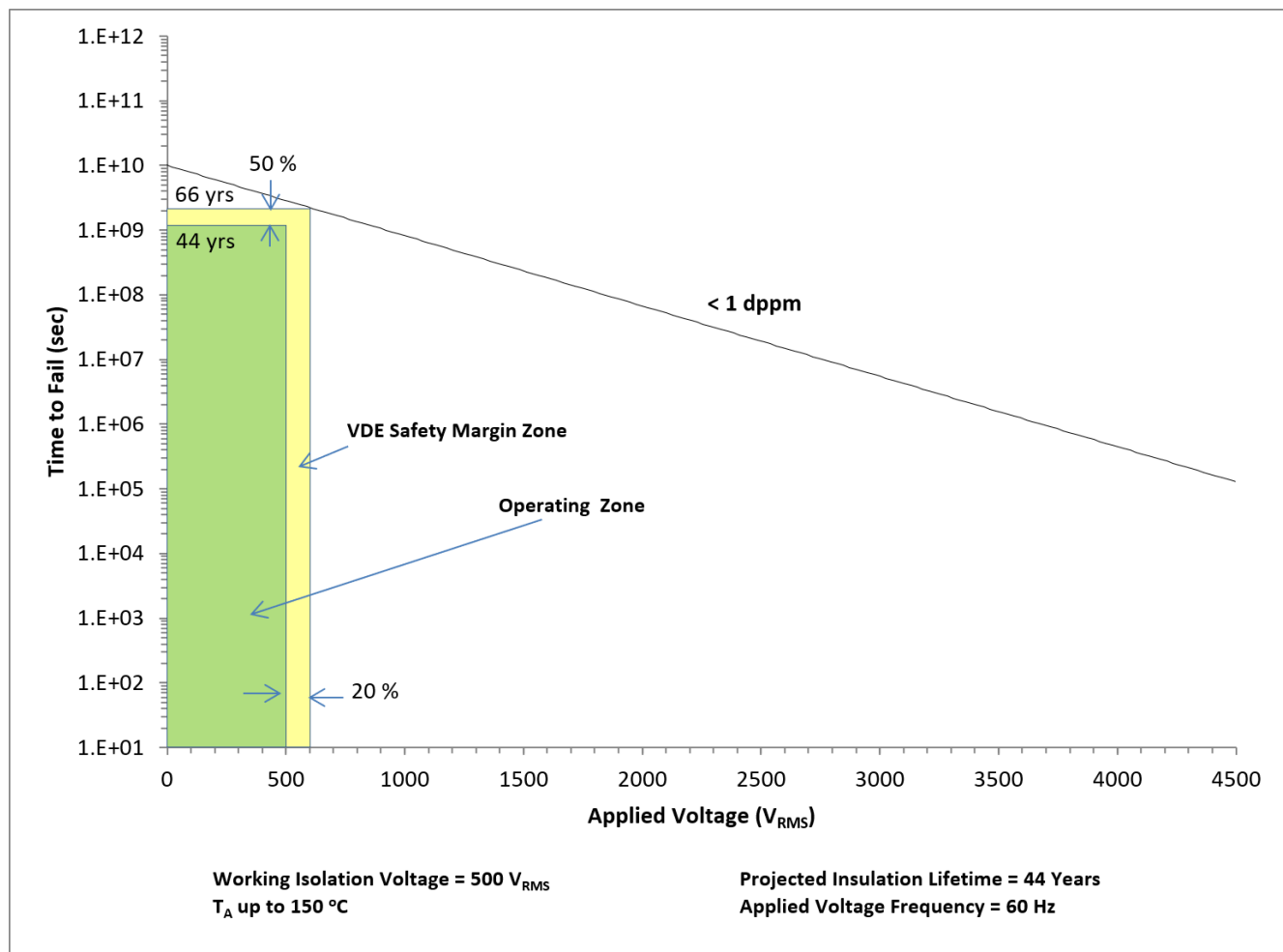
図 9-9. 絶縁寿命予測データ
