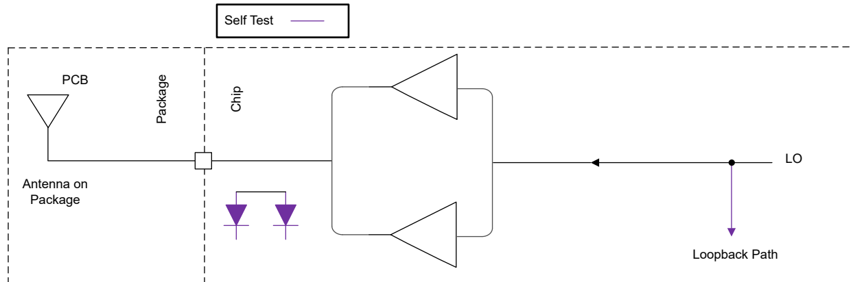
図 8-2. 送信サブシステム (チャンネルごと)
