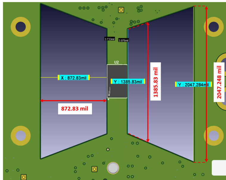
図 7-8. 台形カットアウトと PCB エッジが 0.3mm 未満の大型フォーム ファクタの基板
