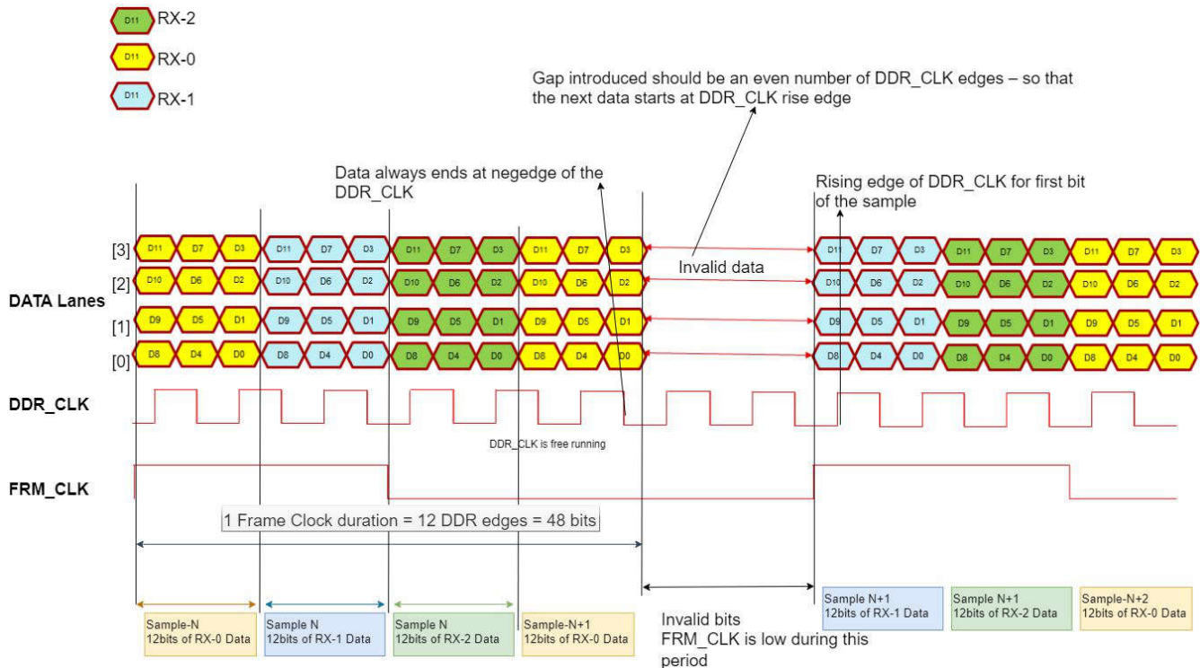
図 7-20. RDIF データ形式
