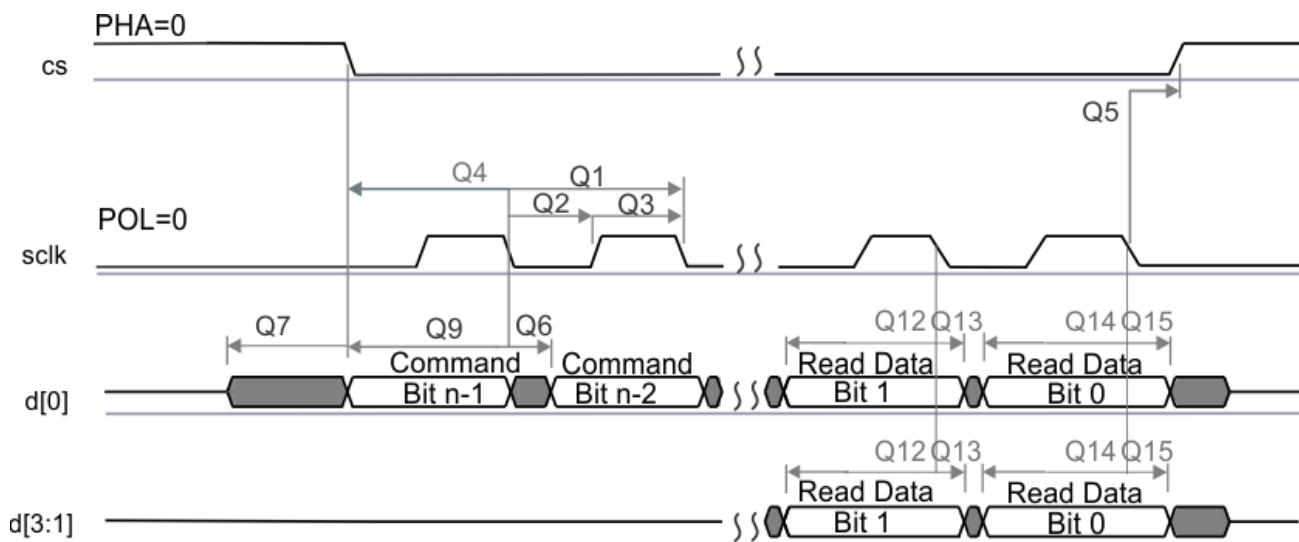
図 7-22. QSPI 読み出し (クロック モード 0)
