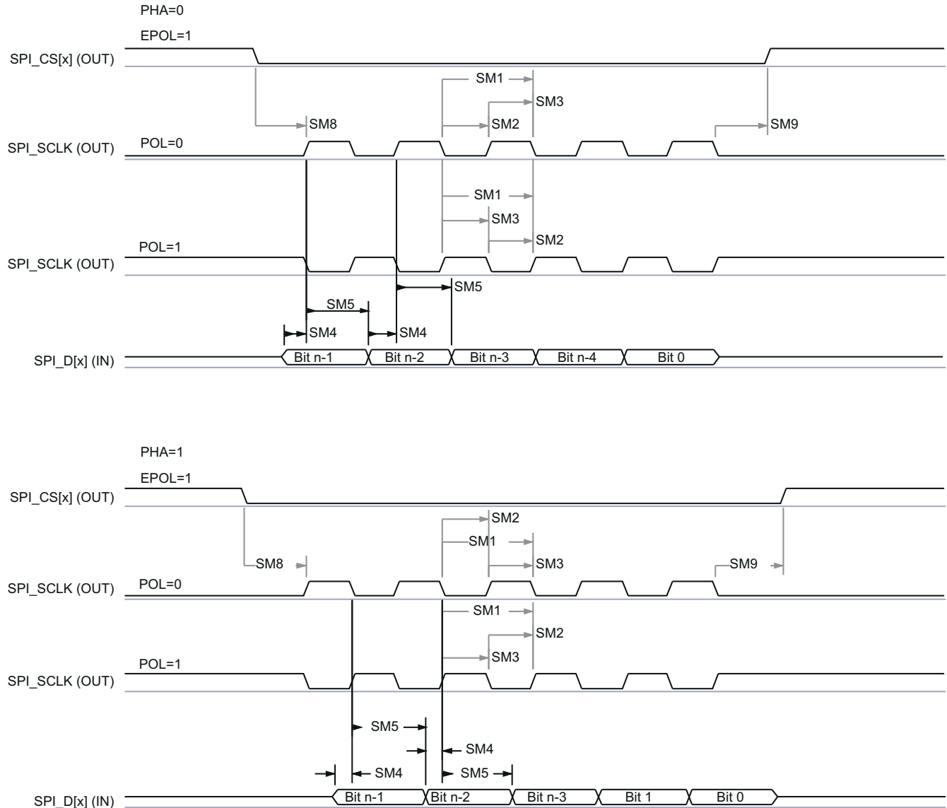
図 7-15. SPI のタイミング - コントローラ モードの受信
