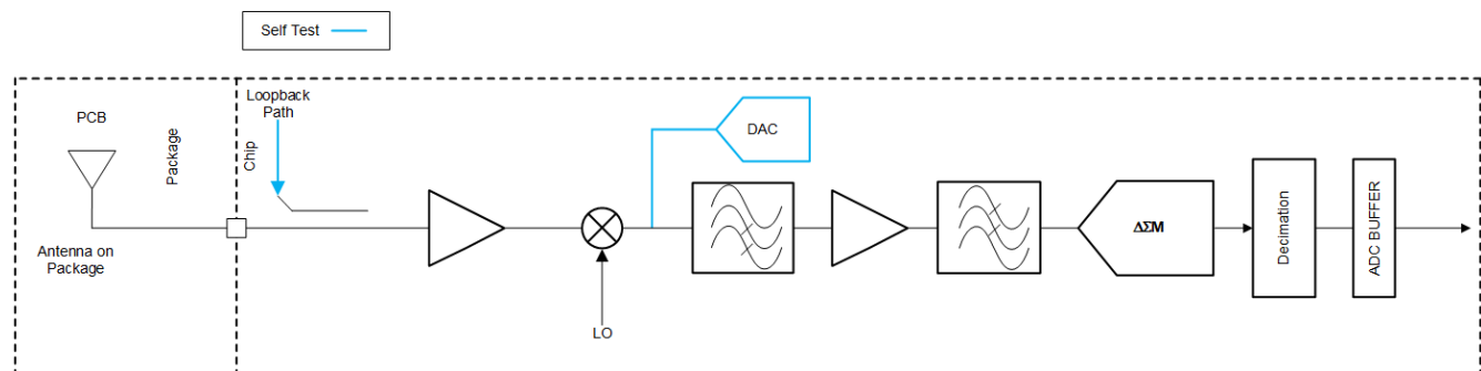
図 8-3. 受信サブシステム (チャンネルごと)
