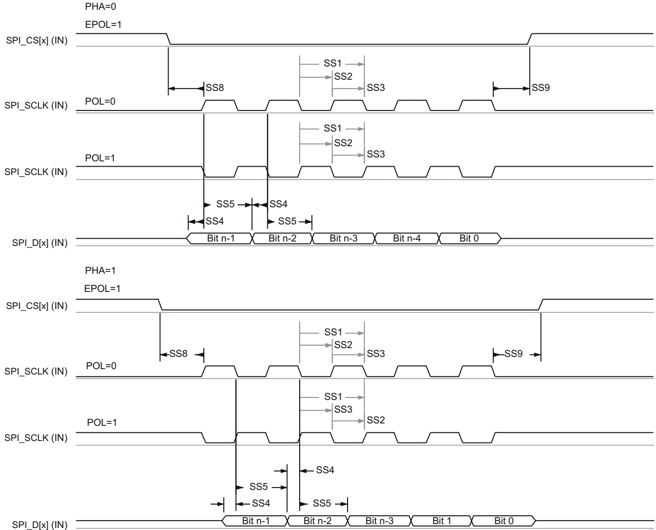
図 7-17. SPI のタイミング - ペリフェラル モードの受信
