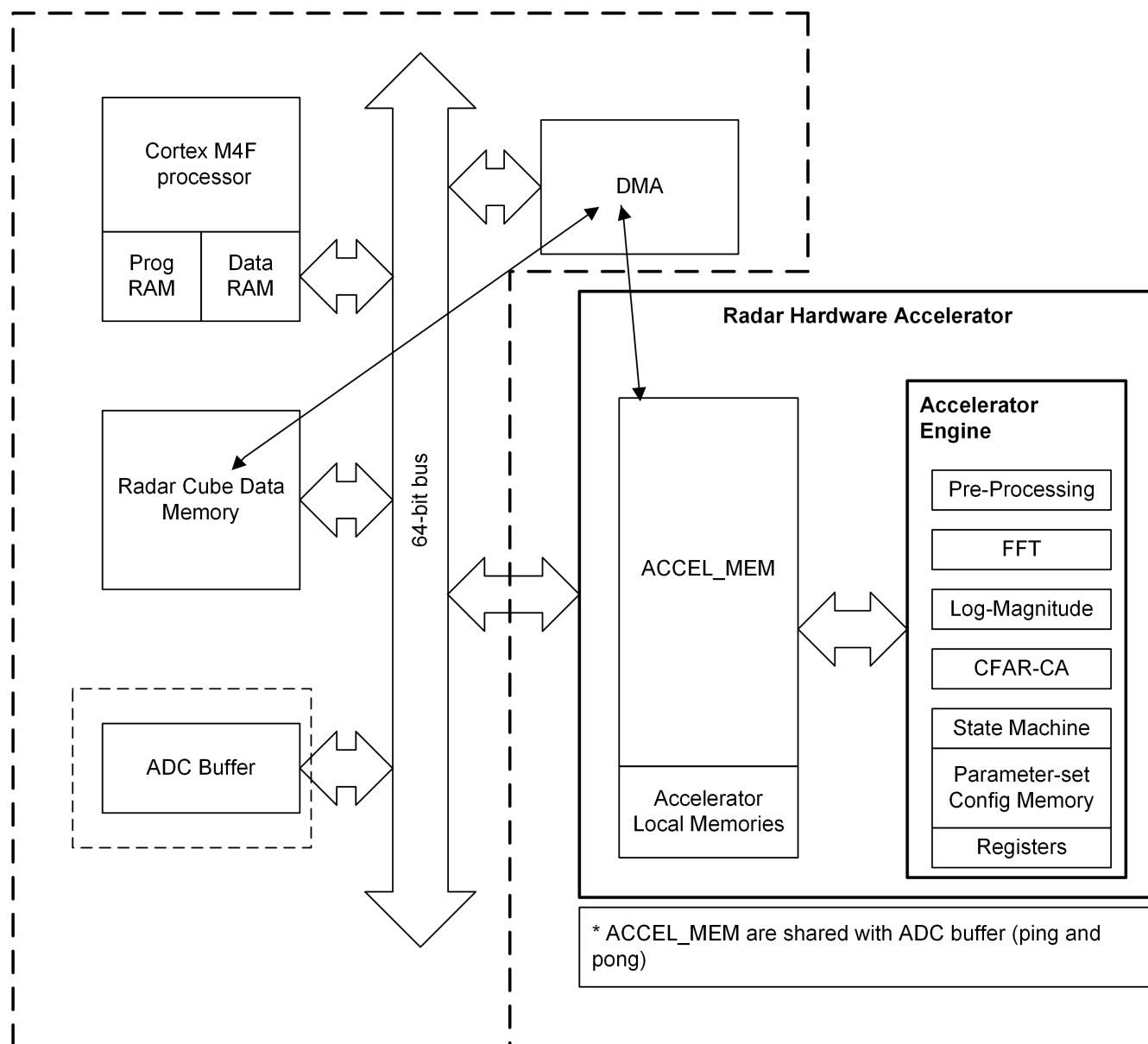
図 8-5. HWA 1.2 の機能ブロック図
