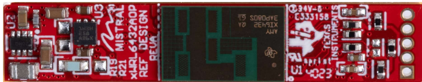
図 7-7. PCB エッジ 0.3mm 未満の IWRL6432AOP リファレンス デザイン
