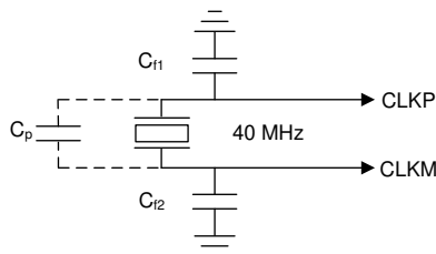
図 7-14. 水晶振動子の実装
