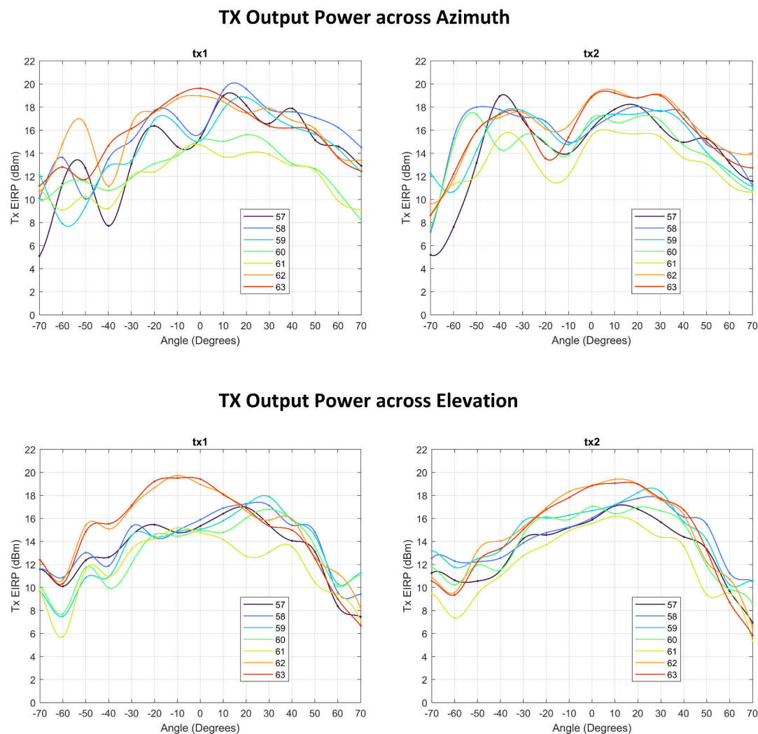
図 7-10. トランスミッタのアンテナ放射パターン
