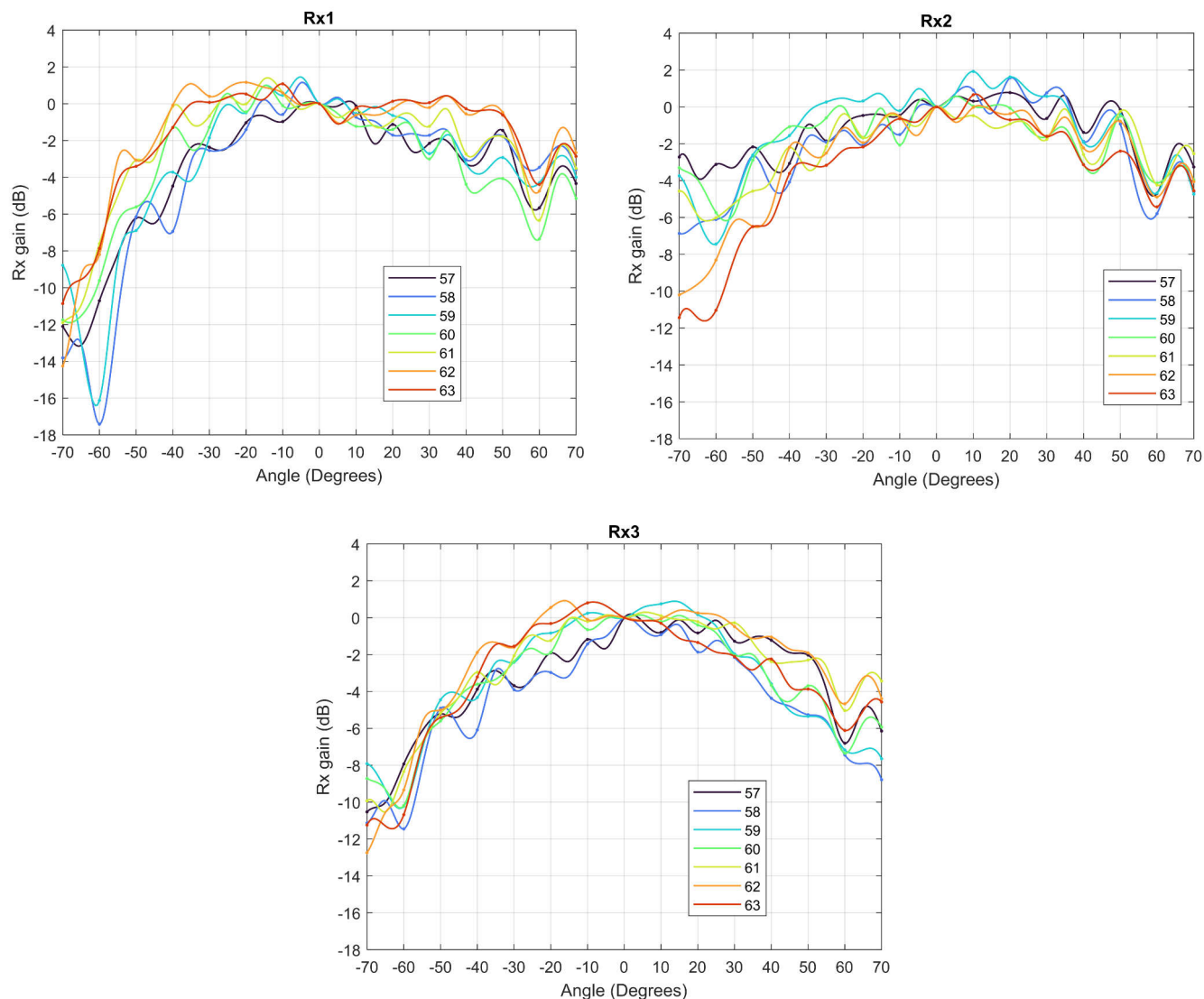
図 7-9. レシーバ ゲイン プロットが照準に正規化されました
