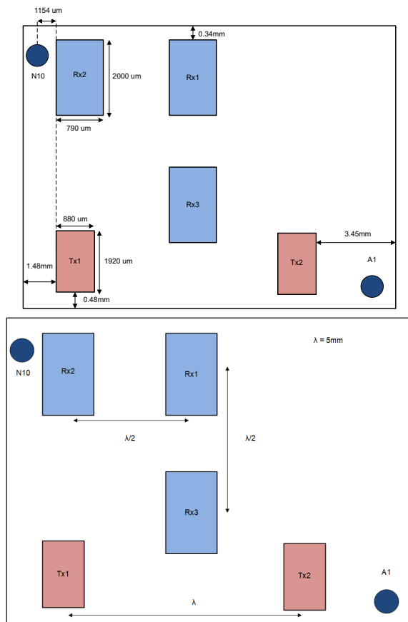
図 7-11. アンテナ位置 (配置と相対間隔)
