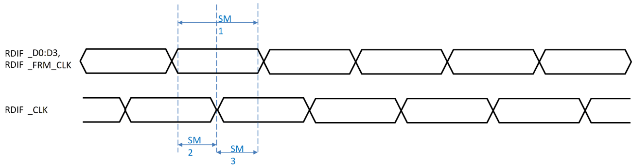
図 7-19. RDIF のタイミング要件
