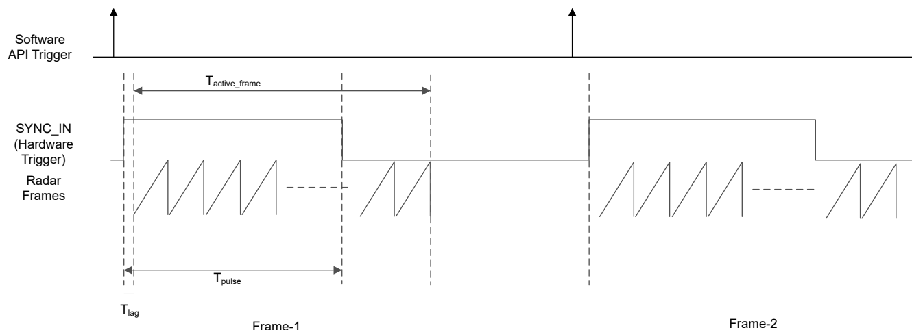
図 7-13. 同期入力ハードウェア トリガ
