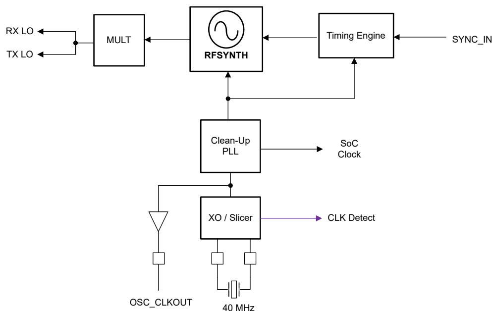
図 8-1. クロック サブシステム
