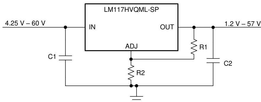
概略回路図
