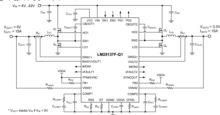
LM25137F-Q1 デュアル出力降圧スイッチングレギュレータ - 概略回路図
