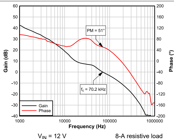
図 9-15. Bode Plot, 5-V Output
