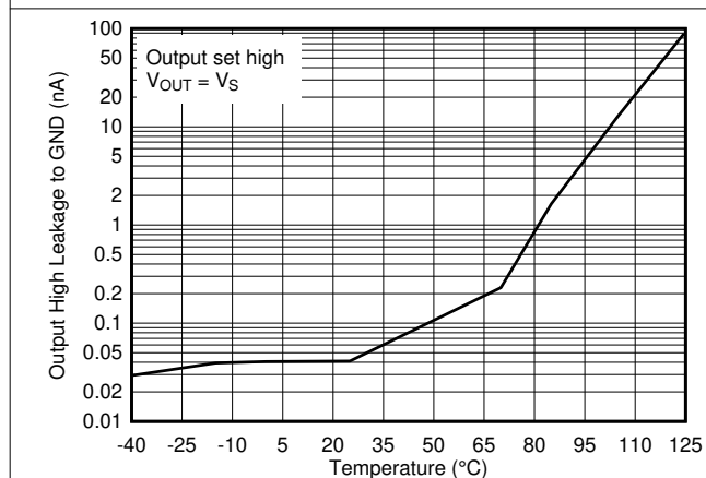
図 5-23. 出力 High リーク電流と温度との関係、5V
