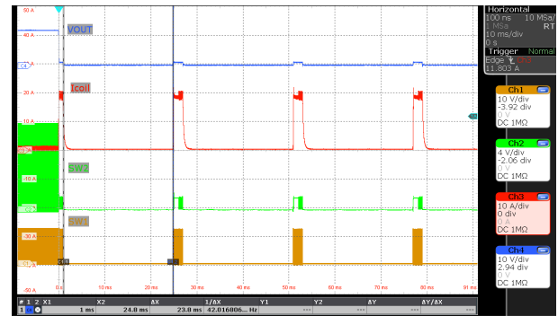
図 10-17. SCP - ヒックアップ保護 ( V_{(VIN)} = 12V , V_{(VOUT)} = 12V I_O = ショート、MODE = VCC2)
