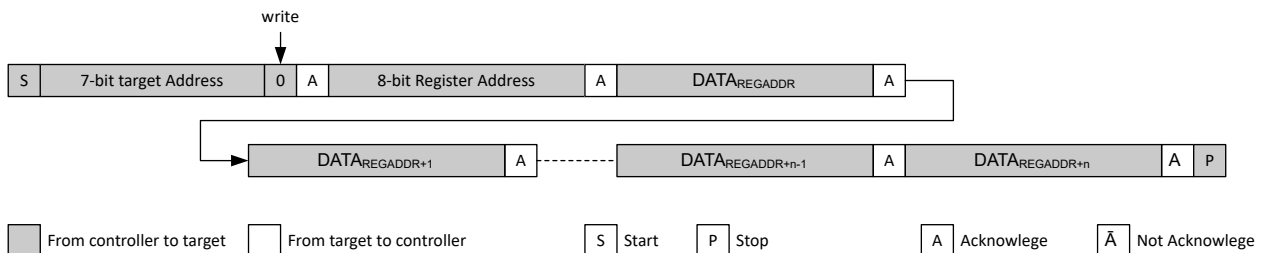
図 8-39. 定義されたレジスタ アドレスから開始されるシーケンシャル WRITE
