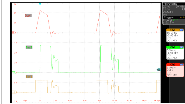
図 10-12. インダクタ電流昇圧モード ( V_{(VIN)} = 12V , V_{(VOUT)} = 12V I_O = 0.05A , MODE = GND )
