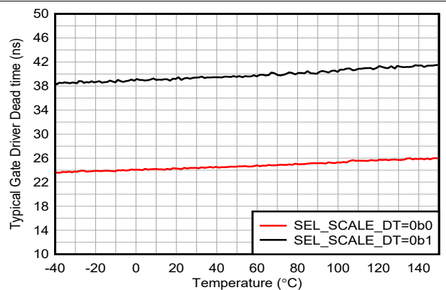
図 6-24. ゲートドライバ遷移 (デッド) 時間とスイッチング周波数との関係 f_{(sw)} = 100\text{kHz} 、SEL_MIN_DEADTIME_GDRV = 0b01、 EN_CONST_TDEAD = 0b0、ローサイド オフ、ハイサイドをオンに します
