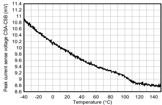
図 6-30. 平均電流制限スレッシュホールド電圧と温度との関係 ILIM_THRESHOLD = 0x14
