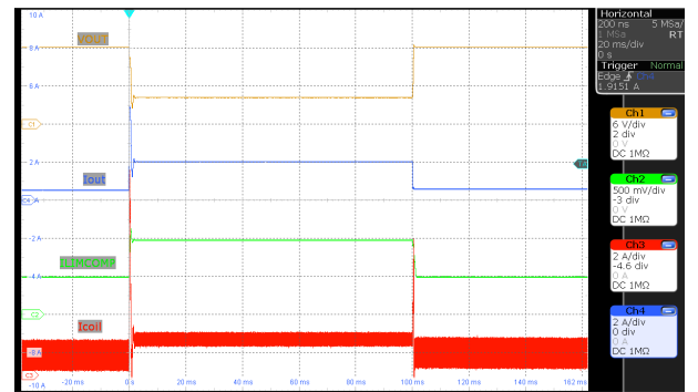
図 10-25. 平均出力電流制限 ( V_{(VIN)} = 6V , V_{(VOUT)} = 12V I_O = 0.5A \leftrightarrow 5A , MODE = VCC2, ILIM_THRESHOLD = 0x28 (2A))
