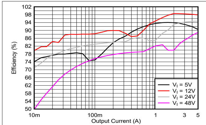
図 10-2. 効率と I_O の関係 (MODE = 0V, V_O = 12V )
