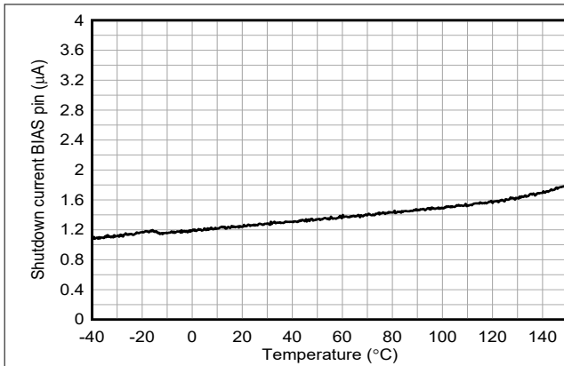
図 6-7. BIAS に流れ込むシャットダウン電流と温度との関係 V_{EN/UVLO} = 0\text{V} 、 V_{(VIN)} = 3.5\text{V} 、 V_{(BIAS)} = 12\text{V}
