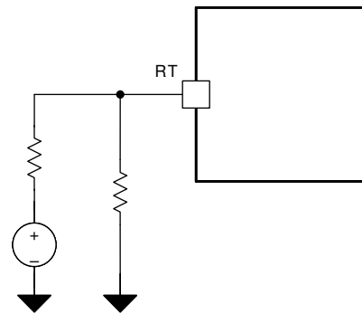
図 8-21. 動的な周波数変更の例
