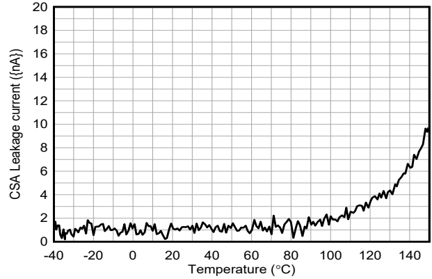
図 6-26. CSA 入力電流と温度との関係
