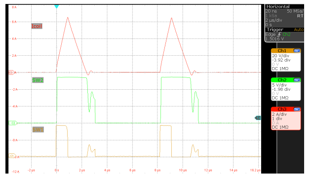
図 10-13. インダクタ電流昇圧モード ( V_{(VIN)} = 36V , V_{(VOUT)} = 12V I_O = 0.05A , MODE = GND )
