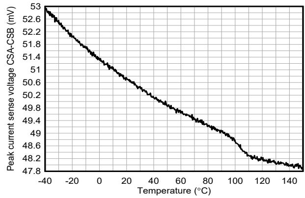
図 6-28. 平均電流制限スレッシュホールド電圧と温度との関係 ILIM_THRESHOLD = 0x64
