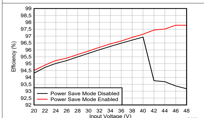
図 10-6. 効率と V_I ( V_O = 48V , I_O = 5A )
