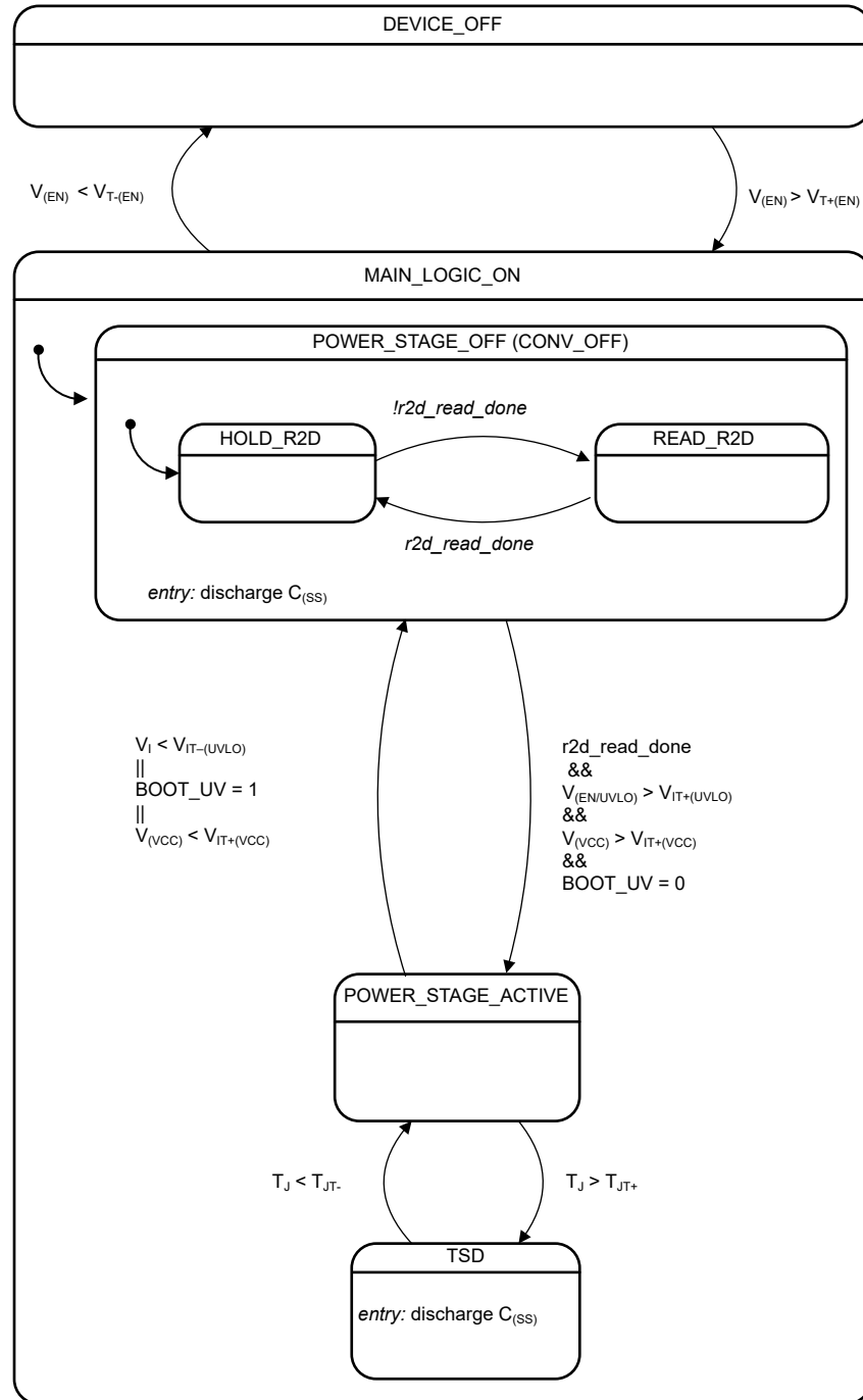
図 8-32. 状態遷移図
