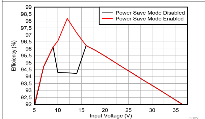
図 10-4. 効率と V_I との関係 ( V_O = 12V , I_O = 5A )
