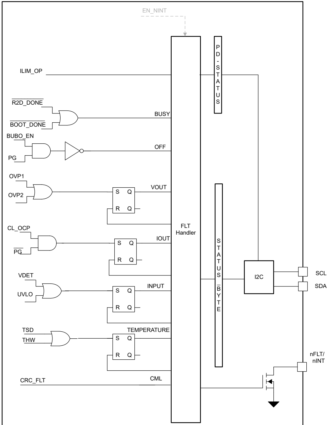
図 8-29. 機能ブロック図フォルトハンドラ
