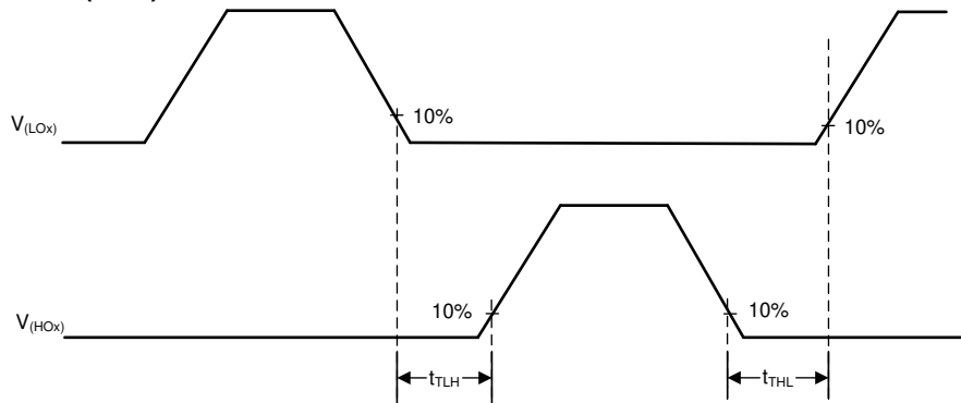
図 7-2. タイミング図ゲート ドライバ t_d
