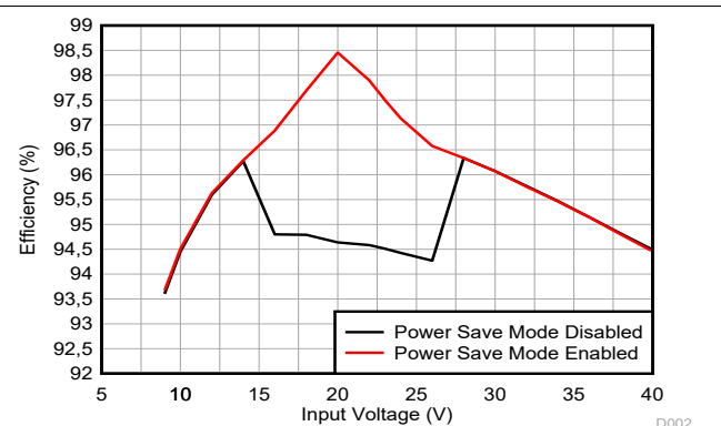
図 10-5. 効率と V_I ( V_O = 20V , I_O = 5A )
