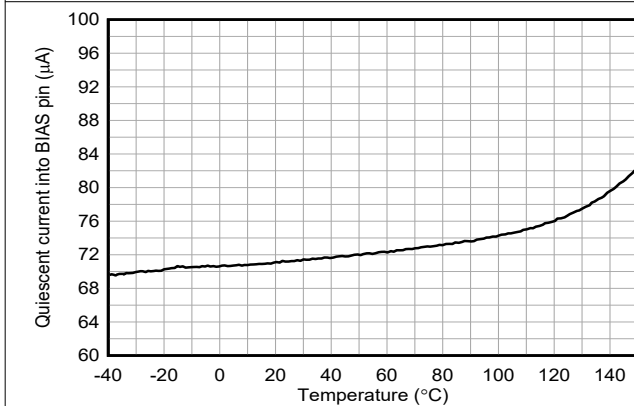
図 6-9. BIAS と BIAS の間の静止電流 V_{(BIAS)} = 12\text{V} 、 V_{(VIN)} = 3.5\text{V}
