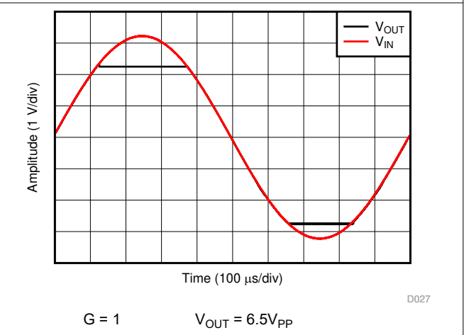
図 6-21. 位相反転なし
