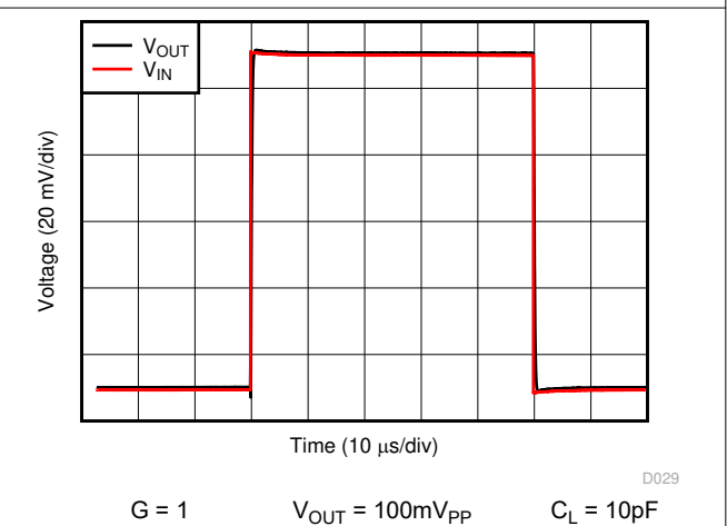
図 6-23. 小信号ステップ応答
