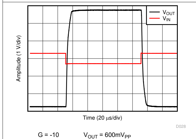
図 6-22. 過負荷からの回復
