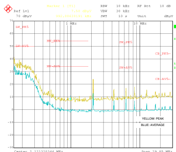
伝導 EMI: V_{OUT} = 5V 、 f_{SW} = 2100\text{kHz}
