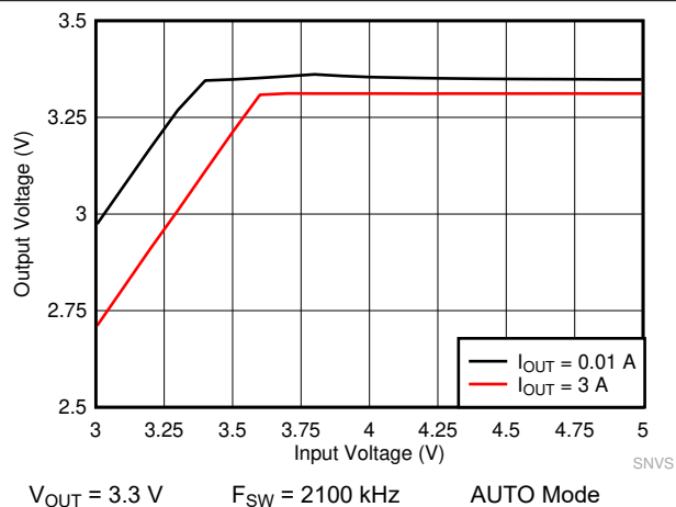
图 9-18. LM61435-Q1 Dropout Curve
