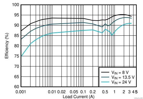
効率: V_{OUT} = 5V 、 f_{SW} = 2200\text{kHz}
