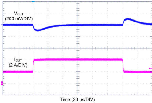
10-25. LM62440-Q1 Load Transient
