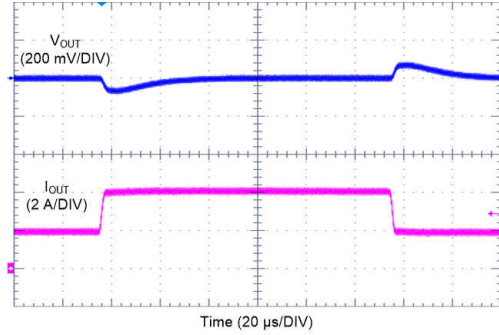
10-24. LM62440-Q1 Load Transient
