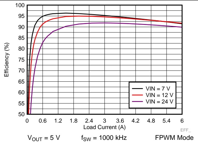
图 36. LM73606 Efficiency
