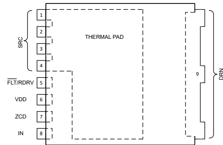
图 5-4. LMG3657R070, TOLL Package (Top View)
