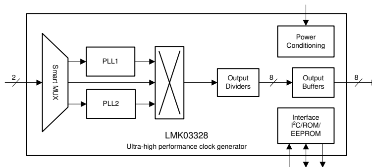
LMK03328 概略ブロック図
