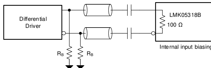
図 8-13. リファレンス (PRIREF/ SECREF) または XO 入力への HCSL (ロード終端)
