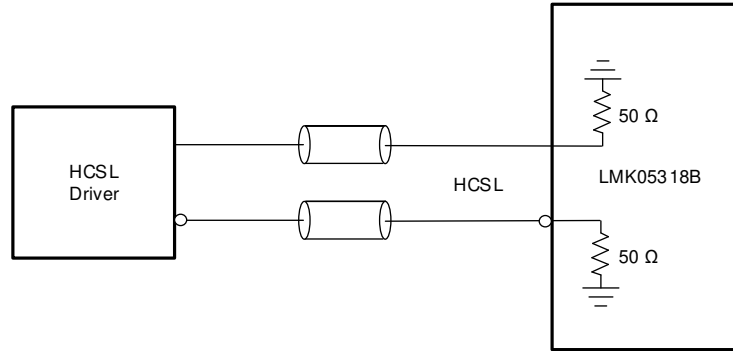
図 8-13. リファレンス (PRIREF/ SECREF) または XO 入力への HCSL (ロード終端)
