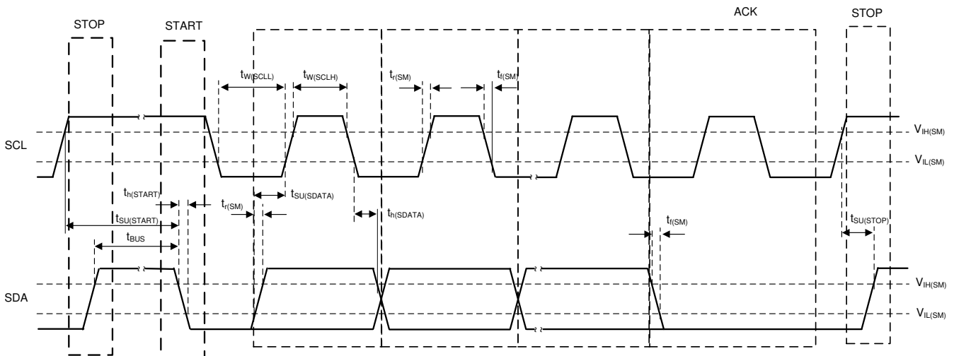
図 6-2. I 2 C のタイミング図
