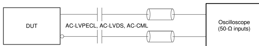
図 7-3. AC-LVPECL、AC-LVDS、AC-CML 出力 AC テスト構成
