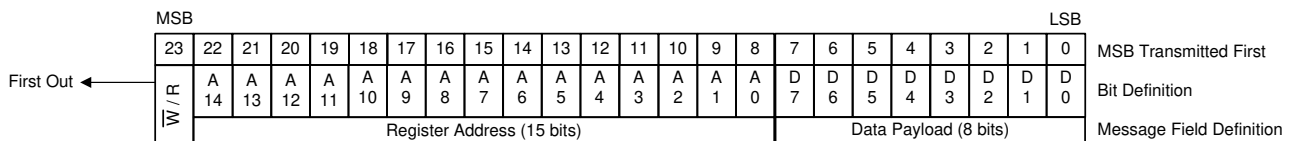
図 8-39. SPI メッセージ形式
