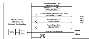
代表的なシステム ブロック図
