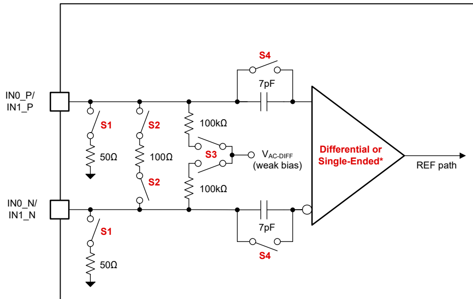
図 7-8. Reference Input Buffer
