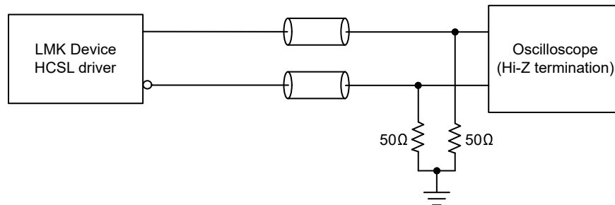
図 6-7. HCSL Output Time Domain Test Configuration
