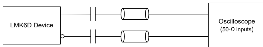
図 7-3. LMK6D 出力テスト構成
