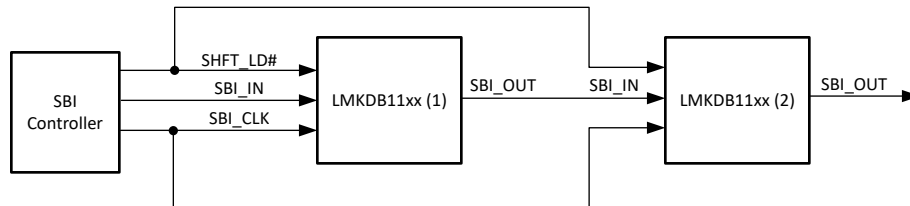
図 8-14. SBI デ이지ーチェーントポロジ
