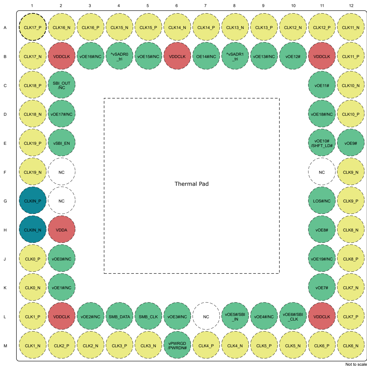
図 5-1. LMKDB1120 および LMKDB1120FS 6mm x 6mm NPP パッケージ 80 ピン TLGA 上面図
