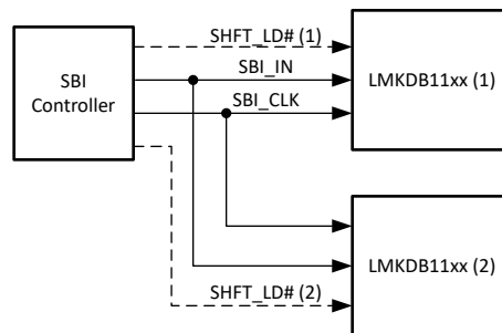
図 8-13. SBI スタート ポロジ
