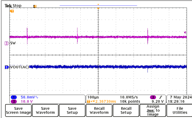
8-16. Output Ripple
