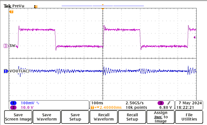
8-17. Output Ripple
