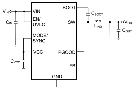
概略回路図
