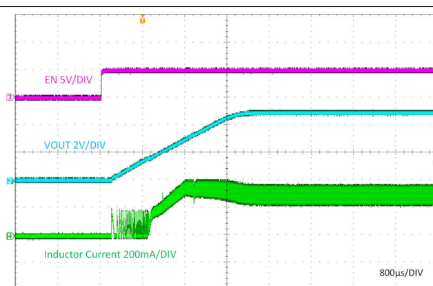
図 8-6. Start-Up by EN
