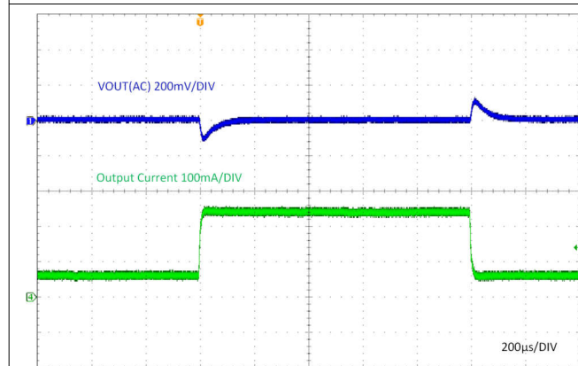
図 8-7. Load Transient (60mA – 240mA)
