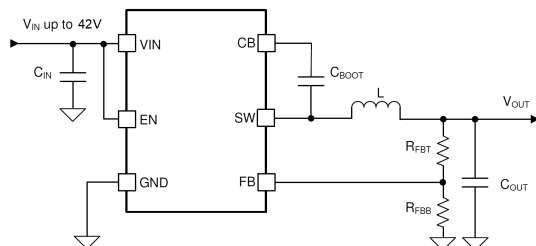
概略回路図
