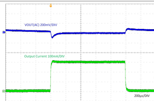
図 8-8. Load Transient (0mA – 300mA)
