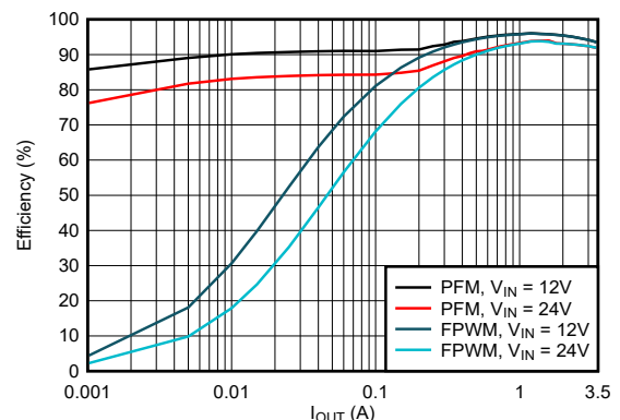
効率と出力電流との関係 V_{OUT} = 5V 、500kHz
