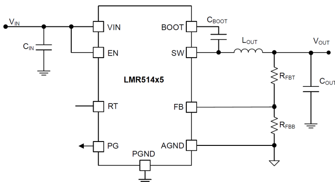
概略回路図
