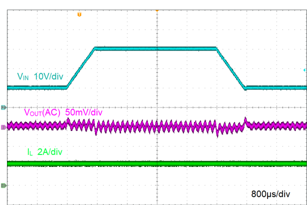
図 8-7. Line Transient
