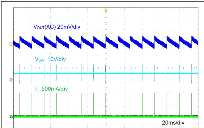
図 8-2. Ripple at No Load
