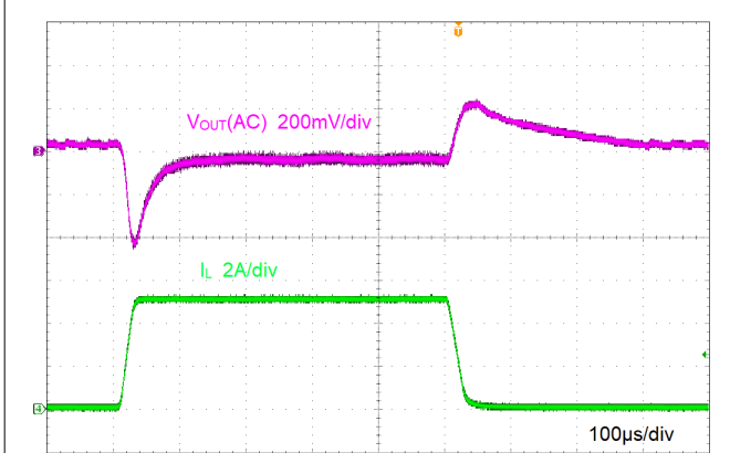
図 8-6. Load Transient
