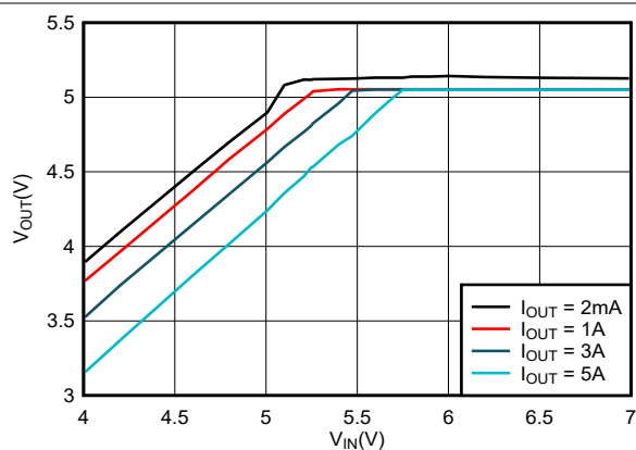
図 6-7. 5V Dropout
