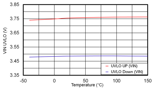
図 6-10. V_{IN} UVLO
