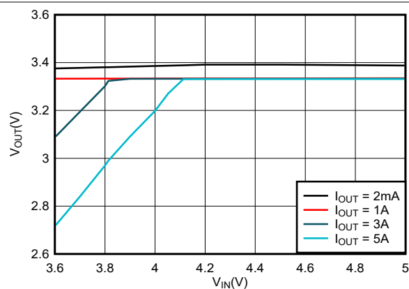
図 6-8. 3.3V Dropout
