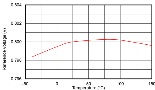
図 6-11. Reference Voltage
