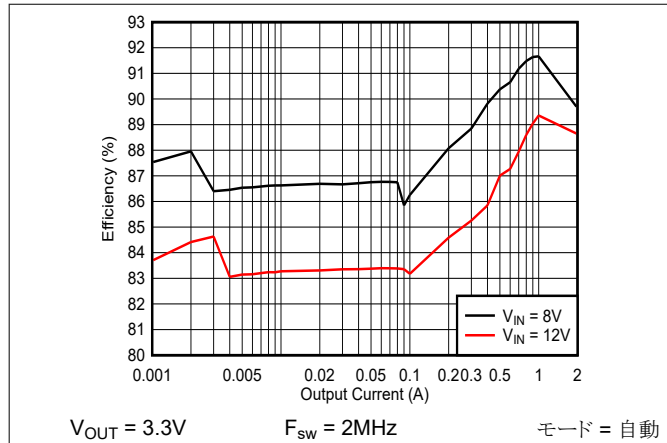
図 8-2. 効率
