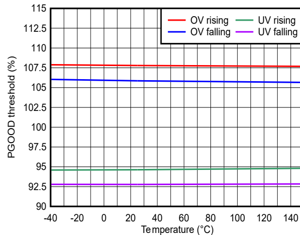
図 6-11. PGOOD スレッシュホールド
