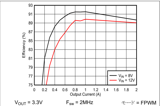
図 8-3. 効率
