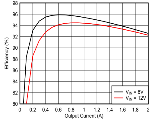
図 8-9. 効率
