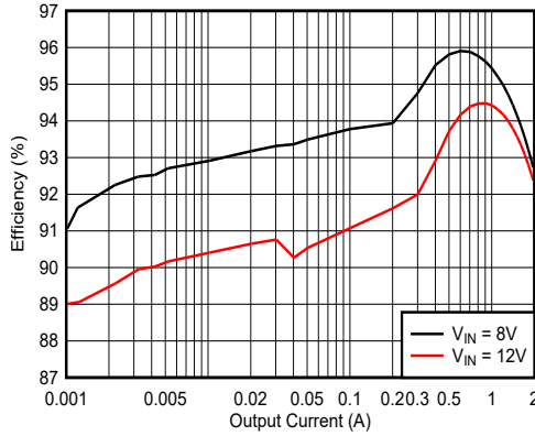
図 8-8. 効率
