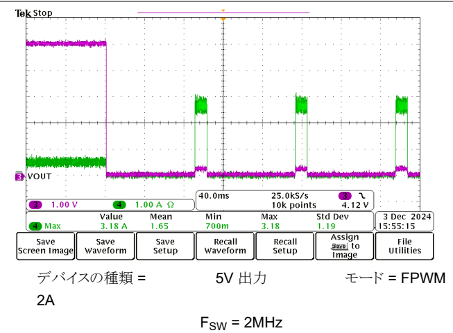
図 8-21. 短絡発生
