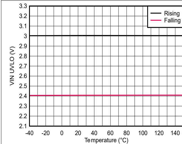
図 6-9. 入力電圧 UVLO 保護 - 「A」バリエーション
