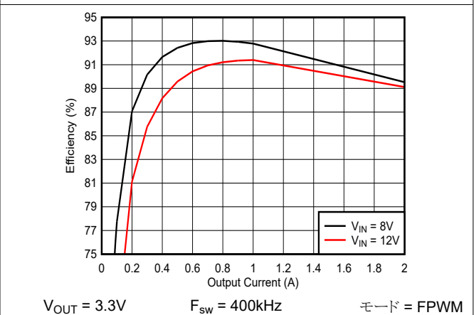
図 8-5. 効率
