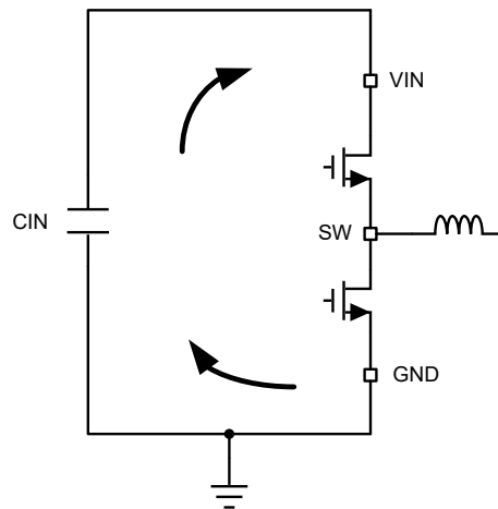
図 8-36. 高速エッジを持つ電流ループ
