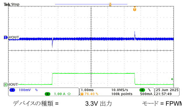
図 8-15. 0A ~ 2A の負荷過渡
