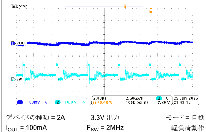
図 8-24. 定常状態波形
