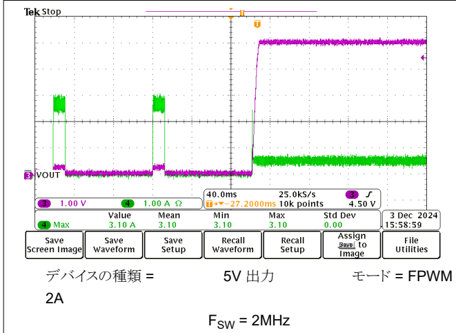
図 8-22. 短絡からの回復
