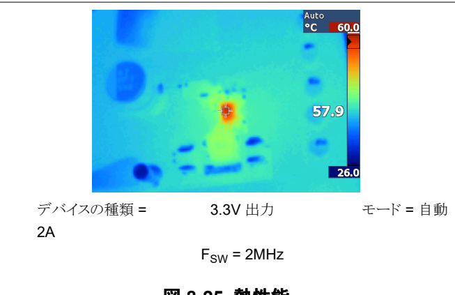
図 8-25. 熱性能
