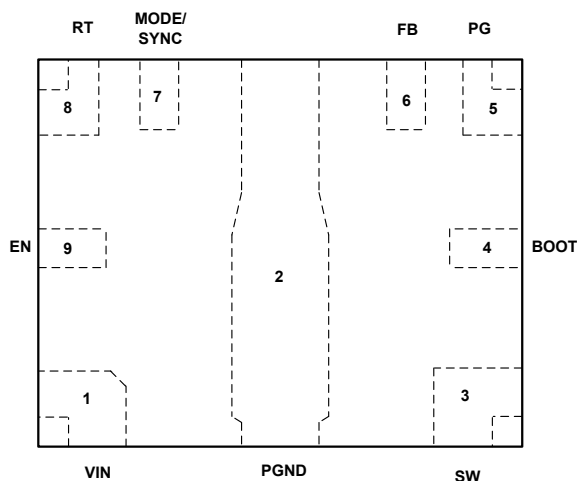
図 5-1. RAK パッケージ 9 ピン WQFN-HR (上面図)
