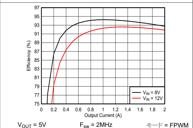
図 8-7. 効率
