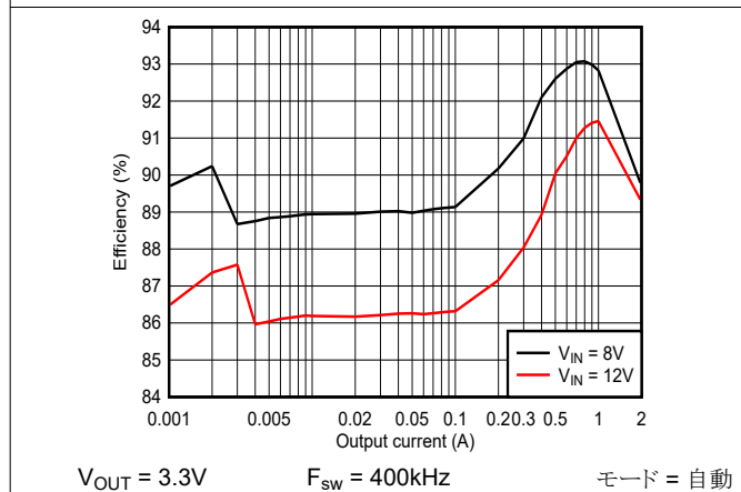
図 8-4. 効率
