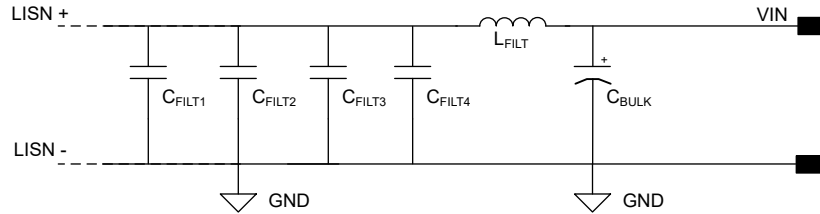
図 8-34. 標準入力 EMI フィルタ回路図
