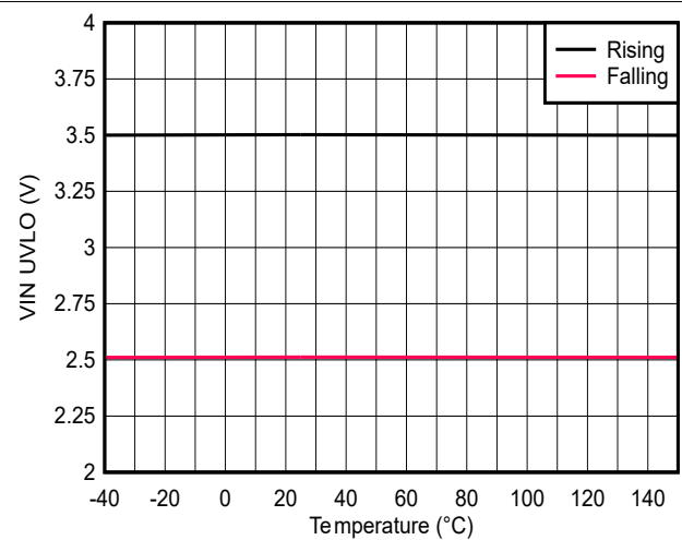
図 6-10. 入力電圧 UVLO 保護 - 「B」バリエーション
