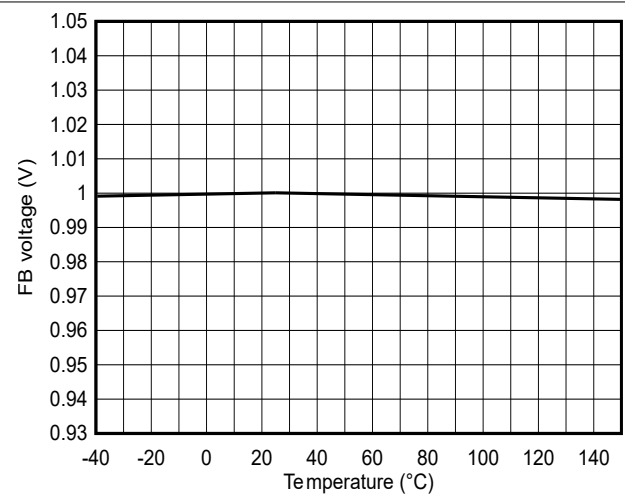
図 6-8. 帰還電圧精度
