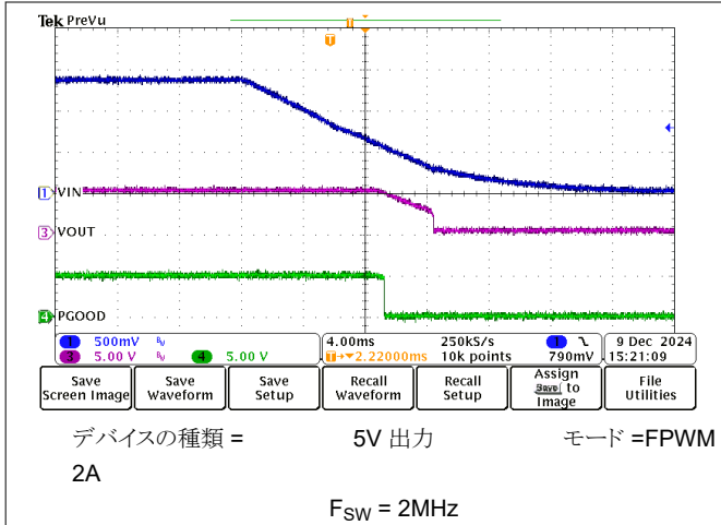
図 8-20. シャットダウン動作
