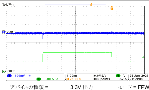
図 8-16. 1A ~ 2A の負荷過渡
