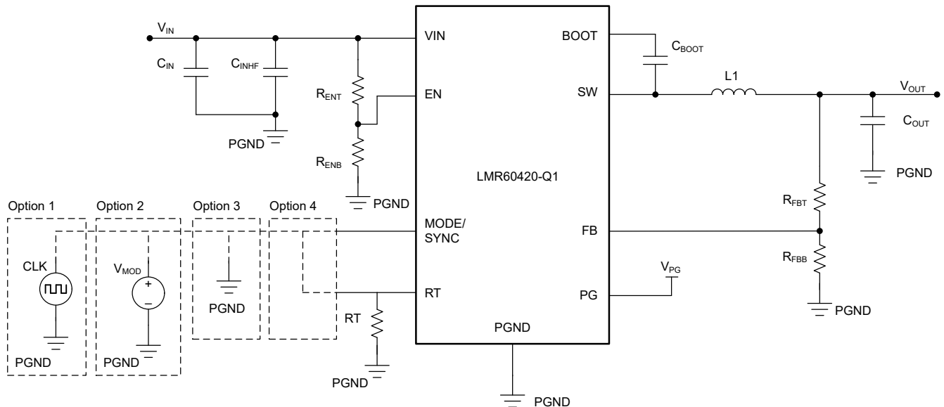
図 8-1. LMR60420-Q1 のリファレンス回路図
