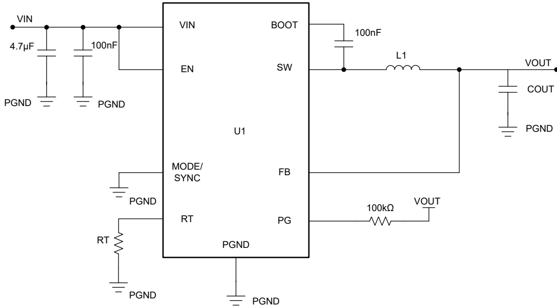
図 8-35. アプリケーション回路例
