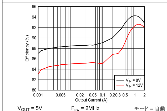
図 8-6. 効率
