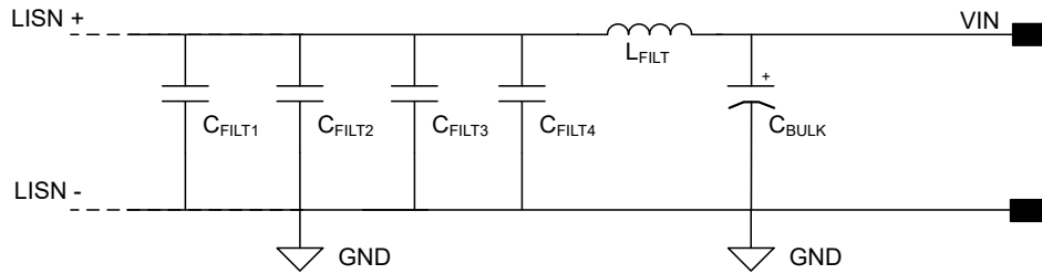
図 8-24. 標準入力 EMI フィルタ回路図
