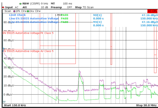
V_{OUT} = 3.3\text{V} F_{SW} = 2\text{MHz} I_{OUT} = 3\text{A} 測定周波数: 150kHz ~ 30MHz
