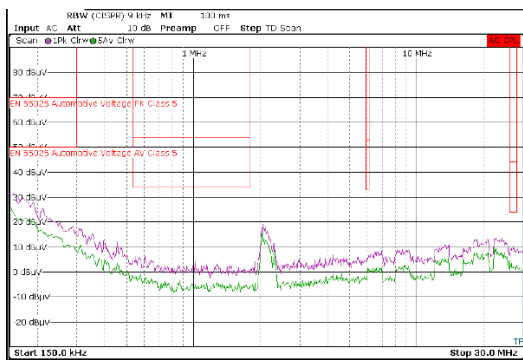
V_{OUT} = 5\text{V} F_{SW} = 2\text{MHz} I_{OUT} = 3\text{A} 測定周波数: 150kHz ~ 30MHz
