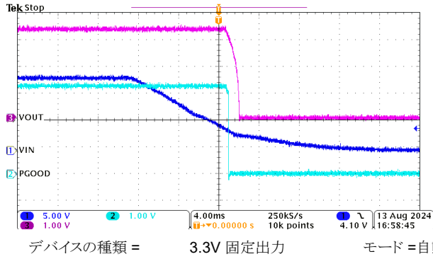
図 8-12. シャットダウン動作
