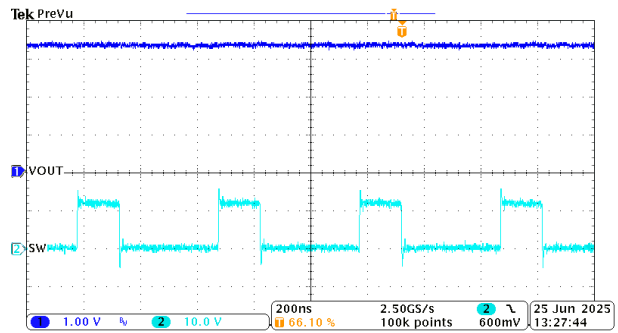
図 8-13. 短絡発生
