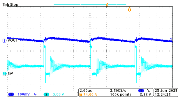
図 8-14. 短絡からの回復
