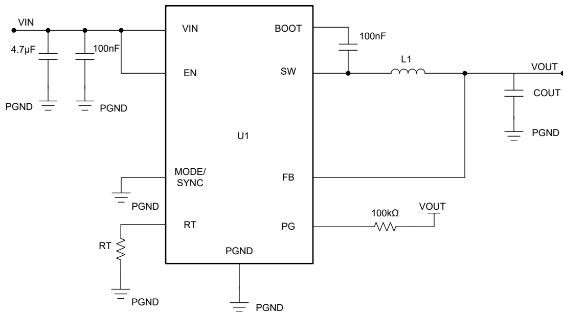
図 8-25. アプリケーション回路例
