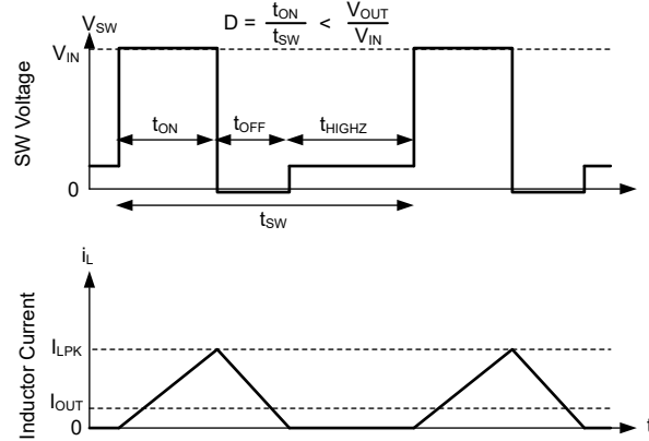
図 7-7. PFM 動作
