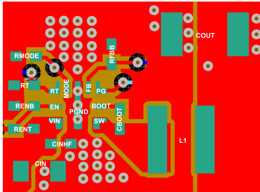
図 8-27. 固定出力バージョン
