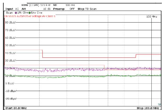
V_{OUT} = 5\text{V} F_{SW} = 2\text{MHz} I_{OUT} = 3\text{A} 測定周波数: 30MHz ~ 108MHz
