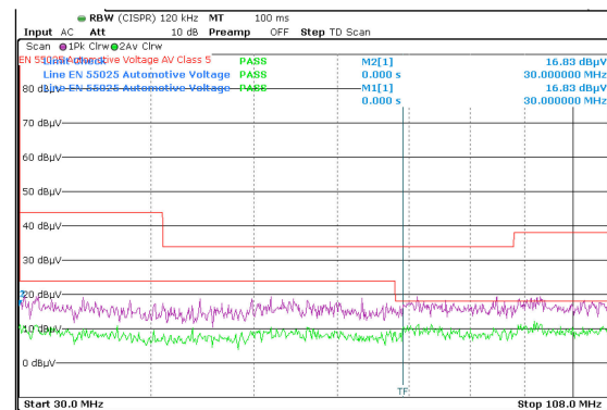
V_{OUT} = 3.3\text{V} F_{SW} = 2\text{MHz} I_{OUT} = 3\text{A} 測定周波数: 30MHz ~ 108MHz
